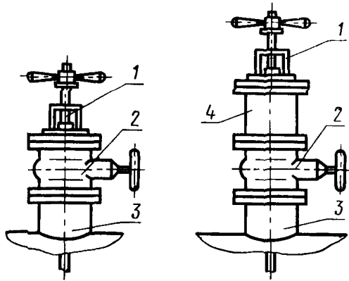
1 — сальниковый ввод; 2 — задвижка (затвор); 3 — патрубок; 4 — шлюзовая камера
