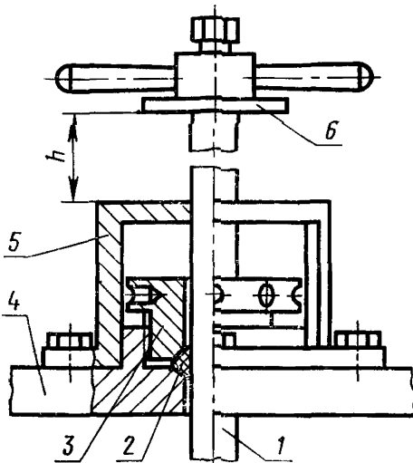
1 — штанга; 2 — набивка сальника, 3 — гайка, 4 — фланец; 5 — скоба; 6 — втулка
