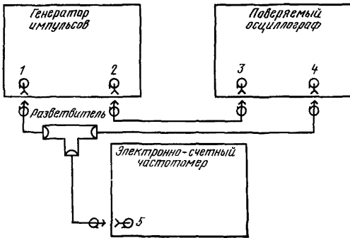
1—выход основных импульсов; 2—выход синхронизирующих импульсов; 3—вход синхронизации; 4—вход усилителя V ; 5—вход частотомера Черт. 7
