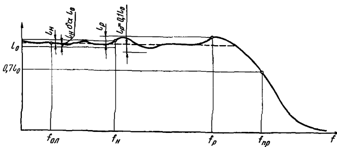
f_{оп} — опорная частота; f_н — нормальный диапазон; f_р — расширенный диапазон; f_{нр} — верхняя граница полосы пропускания; L_0 — значение АЧХ на опорной частоте; L_н — абсолютное значение неравномерности в нормальном диапазоне; L_р — абсолютное значение неравномерности в расширенном диапазоне; \delta_\alpha — относительная погрешность коэффициента отклонения
