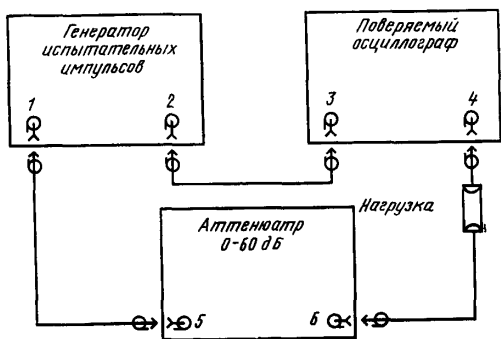
1—выход основных импульсов; 2—выход синхронизирующих импульсов, 3—вход синхронизации; 4—вход усилителя V ; 5—вход аттенюатора; 6—выход аттенюатора
