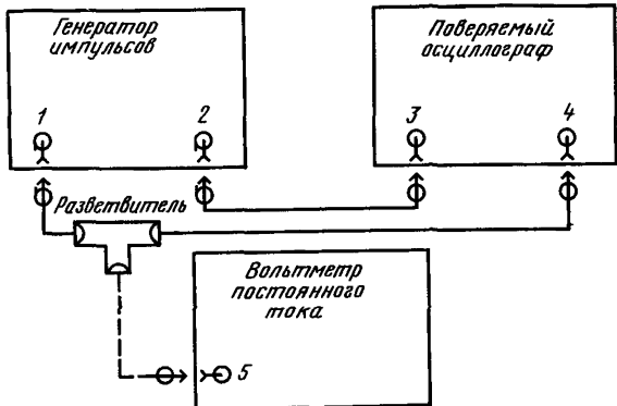
1—выход основных импульсов; 2—выход синхронизирующих импульсов; 3—вход синхронизации; 4—вход усилителя У; 5—вход вольтметра
