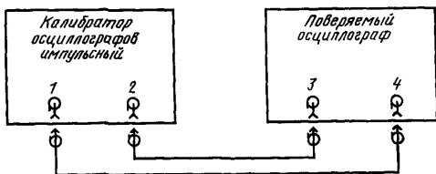
1—выход калибратора временных интервалов; 2—выход синхронизирующих импульсов; 3—вход синхронизации; 4—вход усилителя Y Черт. 8
