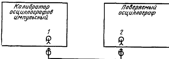
1—выход калибратора напряжения; 2—вход усилителя У.
