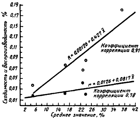
Зависимость сходимости и воспроизводимости от среднего значения величины зольности
