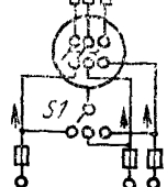
Выключатель по схеме 5
