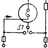
Выключатель по схеме 03
