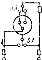
Выключатель по схеме 6
