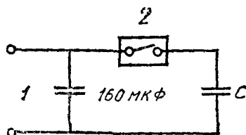
1 — источник питания; 2 — образец Черт. 10
