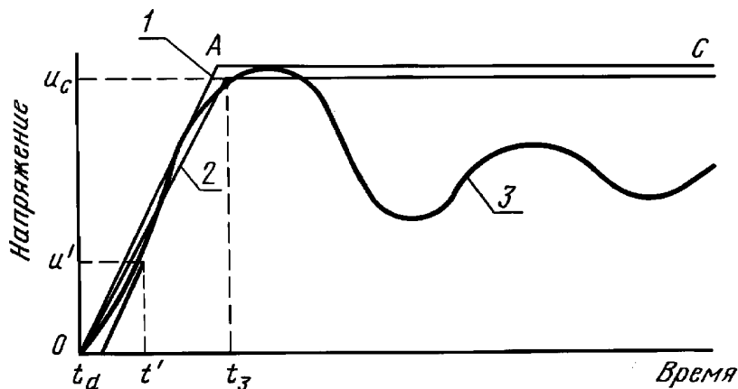
1 — огибающая ПВН; 2 — условная граничная линия ПВН; 3 — собственное ПВН
