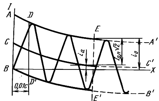
Периодическая и аperiodическая составляющие тока короткого замыкания
