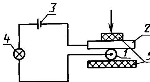
1 — образец; 2 — металлический брусок; 3 — источник питания; 4 — лампочка; 5 — пластинки
