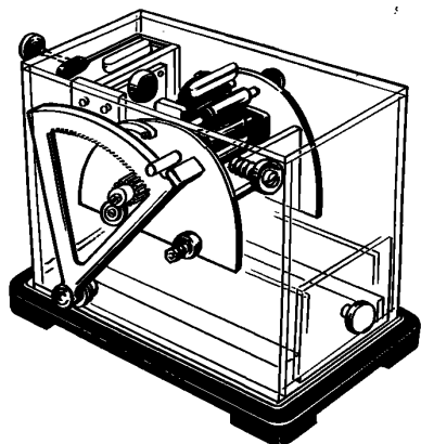
Общий вид прибора «Синазе»
