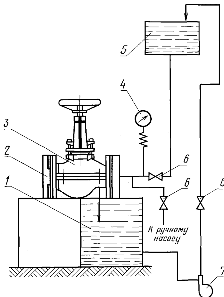
1 — емкость для слива воды; 2 — подвижный зажим; 3 — испытываемое изделие; 4 — манометр; 5 — емкость для воды; 6 — запорный вентиль; 7 — центробежный насос
