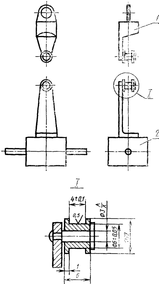
1—верхний зажим; 2—нижний зажим
