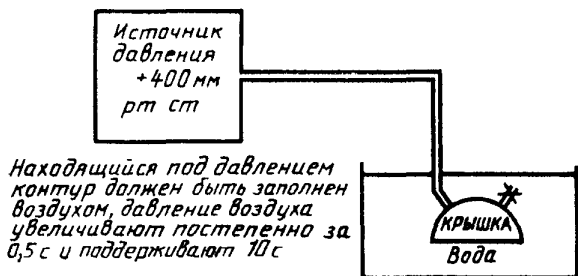
Рисунок 106 — Испытание герметичности диафрагмы (см. 17,101 2)
