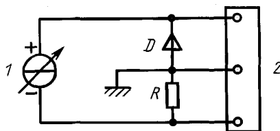
Схема измерения
