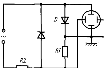
Схема измерения прямого напряжения (метод осциллографа)
