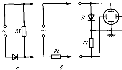
Схема измерения обратного тока (метод осциллографа)
