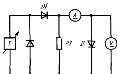
Схема измерения среднего прямого напряжения
