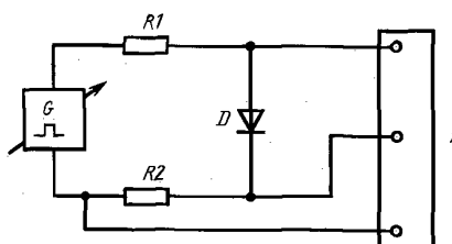
Схема измерения
