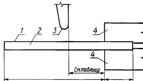
Зажим образца и ударник
