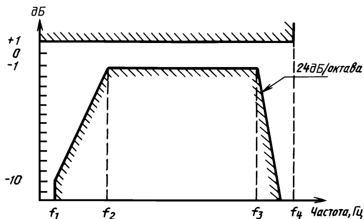
Частотная характеристика измерительной системы
