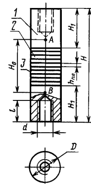
1 — крепежная бобышка; 2 — пластинка; 3 — клеевой слой
