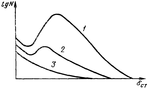
1—высокопрочные эластомеры, кристаллизующиеся при растяжении; 2—высокопрочные наполненные некристаллизующиеся резины, например, из бутадиен-стирольного каучука, 3—малопрочные ненаполненные резины Черт. 2
