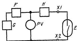
G — источник напряжения; F — защитное устройство; PV — вольтметр; H — индикатор пробоя; E — испытуемый геркон; X1, X2 — клеммы подключения геркона
