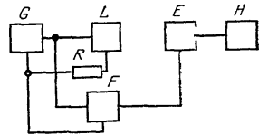
G — генератор прямоугольных импульсов тока; L — измерительная катушка; R — калибровочный резистор; E — испытываемый геркон; H — источник тока; F — устройство измерения времени
