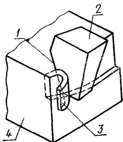
1—режущая кромка; 2— лезвие; 3—стружка; 4—за- готовка
