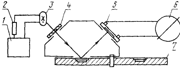
1—стабилизатор напряжения Б 2—2; 2 дроссель, 3—бака терцидная лампа ДБ 15; 4—стеклянная пластинка, не пропускающая излучение с длиной волны 253,7 нм, 5—фотоэлемент селеновый с корригирующим фильтром ФЭС-10, 6—гальванометр типа М 195/2; 7—поворотный диск с кюветами для люминофора
