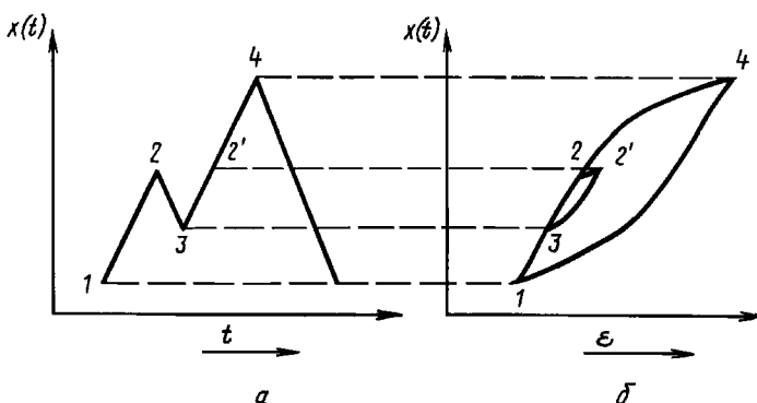
а — фрагмент процесса нагружения; б — диаграмма «напряжение—деформация»
