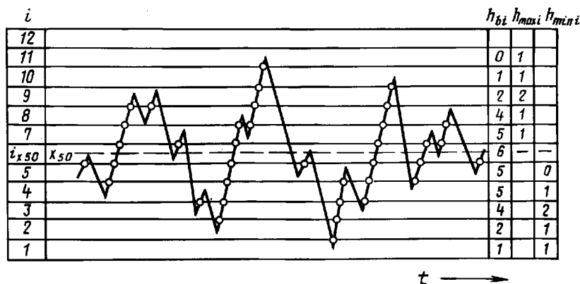
Распределения, полученные по методу пересечений
