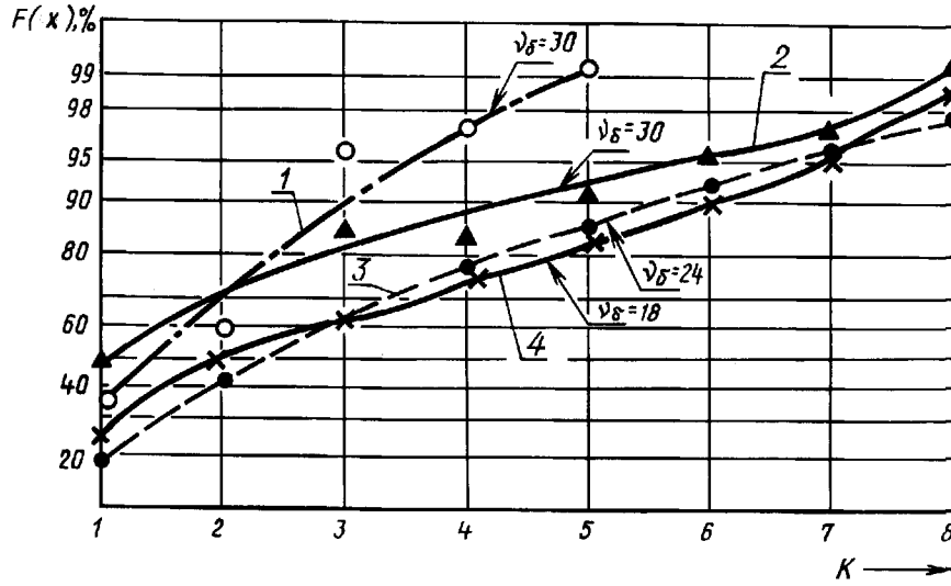
1 — метод размахов; 2 — метод «дождя»; 3 — метод экстремумов; 4 — метод пересечений
