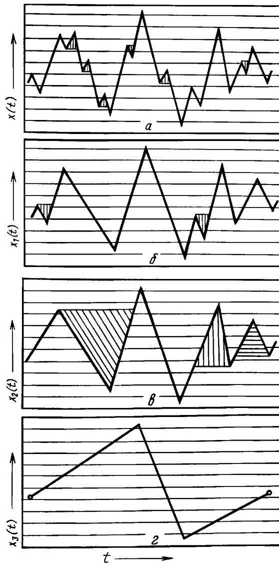
Схематизация по методу полных циклов
