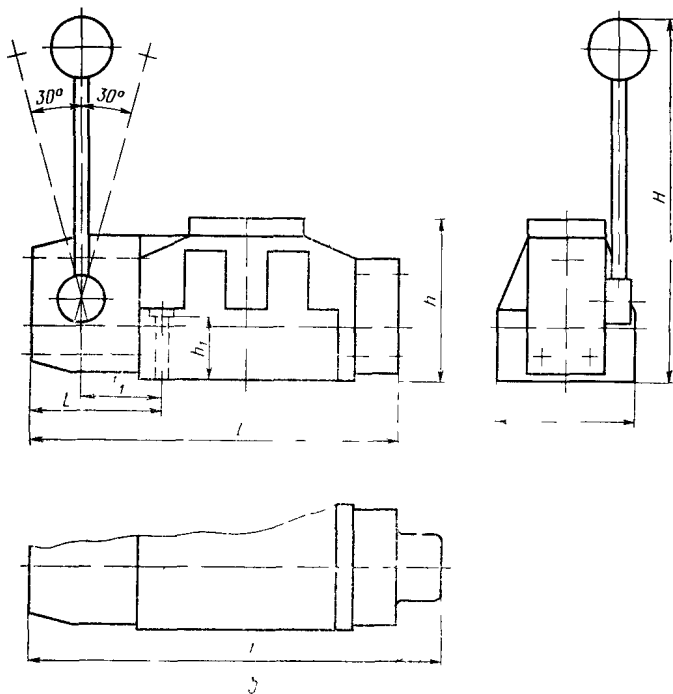
a — трехпозиционный; b — двухпозиционный
