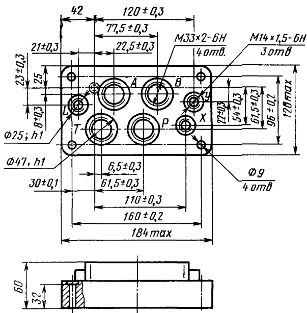
Масса 7,6 кг Черт. 3
