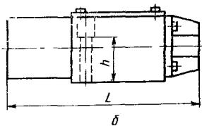
а — с двумя гидроголовками; б — с одной гидроголовкой
