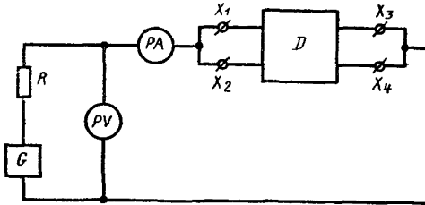
РА—измеритель тока; X_1 , X_2 —входные контакты; D —измеряемый прибор, X_3 , X_4 —выходные контакты; R —защитный резистор, PV —измеритель напряжения; G —генератор тока
