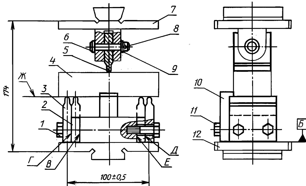
Схема приспособления для испытания на изгиб
