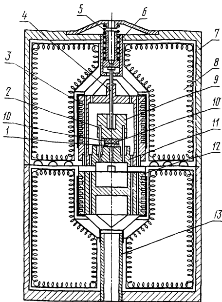
1 — тепломер; 2 — термопара; 3 — эластичная оболочка; 4 — прижим; 5 — пружина; 6 — входной патрубок; 7 — корпус; 8 — теплозащитная оболочка; 9 — стержень; 10 — образец; 11 — основание; 12 — нагревательный блок; 13 — выходной патрубок.
