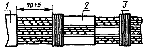
1 — электрический соединитель; 2 — бирка; 3 — бандаж
