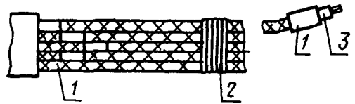
1 — бирки; 2 — бандаж; 3 — наконечник
