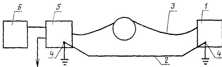
Расположение оборудования при измерении напряжения радиопомех
