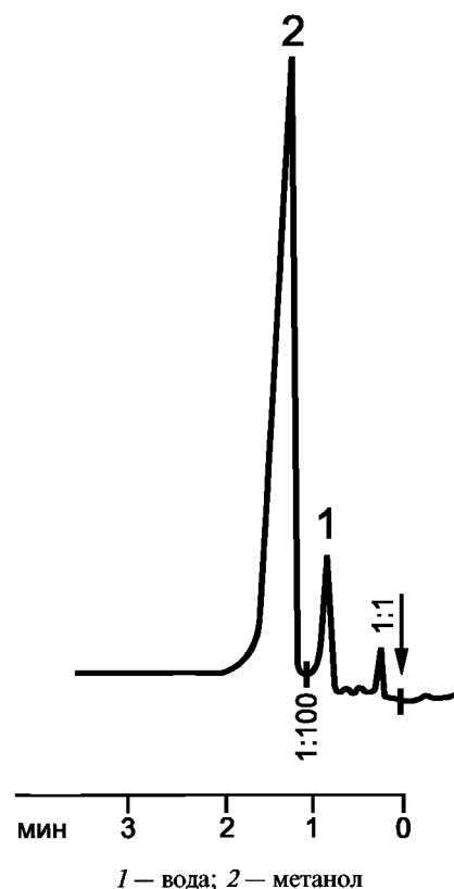
Рисунок Б.1 — Типовая хроматограмма технического метанола
