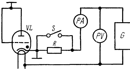
R —резистор; S —выключатель; PA —измеритель тока; PV —измеритель напряжения; VL —испытываемый тиратрон; G —источник постоянного напряжения.
