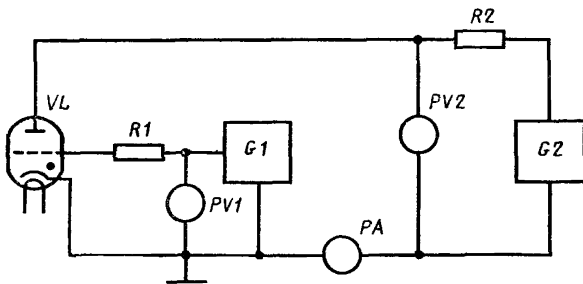
R1, R2 —резисторы; PV1, PV2 —измерители напряжения, PA —измеритель тока; VL —испытуемый тиратрон; G1, G2 —регулируемые источники напряжения
