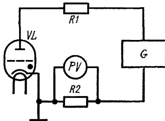
R1 —резистор, R2 —измерительный резистор, PV —измеритель напряжения, VL —испытуемый тиратрон; G —источник напряжения
