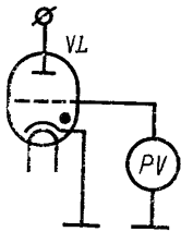
PV —измеритель напряжения, VL —испытуемый тиратрон
