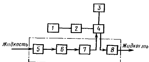
Блок измерения
