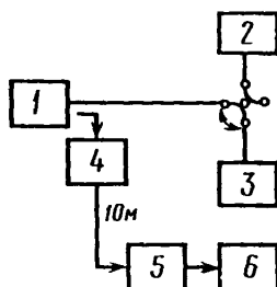
1—радиопередатчик; 2—антенна; 3—эквива- лент антенны по п. 3.2.3; 4—направленный ответ- витель по п. 3.2.4; 5—фильтр по п. 3.2.7; 6—селективный вольт- метр по п. 3.2.12
