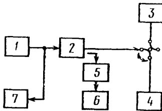
1—генератор сигналов НЧ по п. 328, 2—радиопередатчик, 3—антенна, 4—эквивалент антенны по п. 323, 5—направленный ответвитель по п. 324, 6—девиометр по п. 3210, 7—вольтметр НЧ по п. 329
