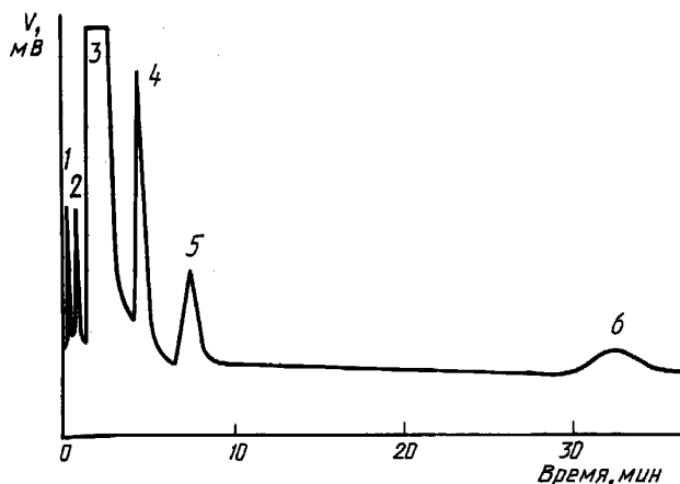
Типовая хроматограмма этиленгликоля с использованием колонки II
