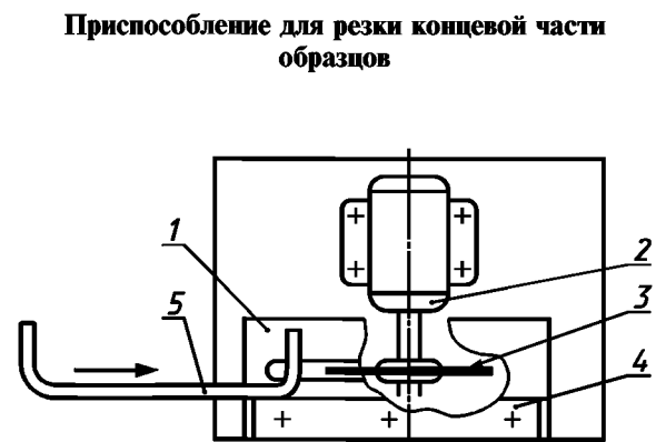
1 — стол; 2 — электродвигатель мощностью 300 Вт; 3 — отрезной диск на специальной бакелитовой основе (электрокорунд белый); 4 — упор; 5 — образец проволоки
