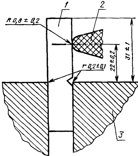
1 — образец; 2 — маятник; 3 — зажим
