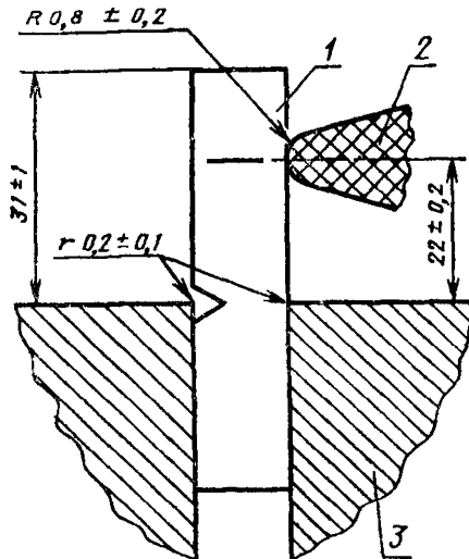
1 — образец; 2 — маятник; 3 — зажим
