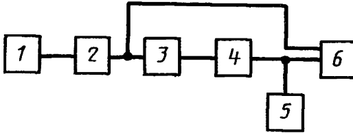
1—генератор 3Ч; 2—датчик испытательных сигналов; 3—генератор сигнала ВЧ; 4—приемник; 5—эквивалент нагрузки; 6—осциллограф
