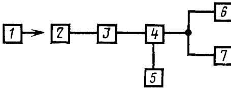
1—электронно-счетный частотомер; 2—генератор сигналов; 3—согласующее устройство (эквивалент антенны); 4—приемник; 5—головные телефоны; 6—эквивалент нагрузки; 7—вольтметр переменного тока
