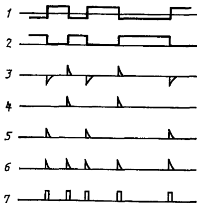
1—входной сигнал; 2—сигнал после формирователя; 3—сигнал на выходе дифференцирующей цепи; 4—неинвертируемые положительные импульсы; 5—сигнал на выходе инвертора; 6—сигнал на входе мультивибратора; 7—выходные импульсы
