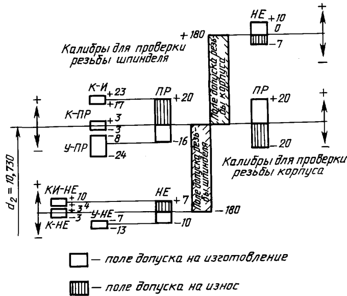
Схема расположения полей допусков среднего диаметра калибров и контракалибров (предельные отклонения в мкм)
