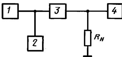
Схема измерения напряжения сигнала с частотой (800 \pm 50) Гц и пределов регулировки уровня сигнала на входах телефонных каналов
