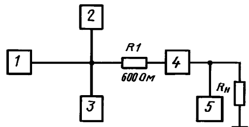
Схема измерения неравномерности частотной характеристики затухания
