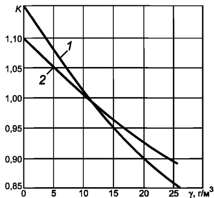
Изменение коэффициента K в зависимости от абсолютной влажности воздуха
