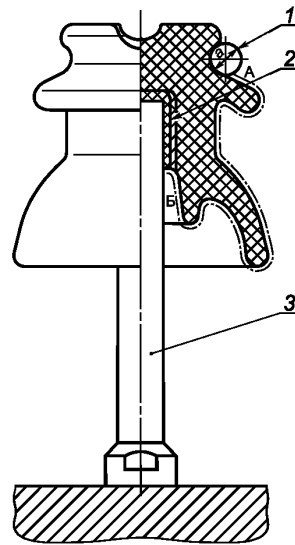
1 — провод; 2 — уплотнитель; 3 — штырь
