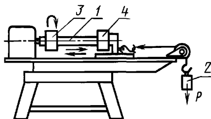
1 — испытуемый образец; 2 — натяжное устройство; 3 — вращающийся зажим; 4 — зажим, имеющий возвратно-поступательное перемещение
