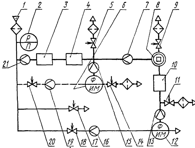
Принципиальная схема установки для контроля фильтрующих коробок по коэффициенту прорыва масляного тумана
