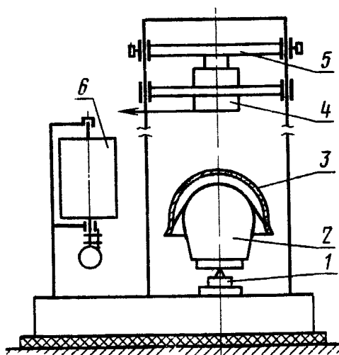
1—сидонизмерительный датчик; 2—макет головы; 3—каска; 4—ударник; 5—каретка; 6—фиксатор прогиба
