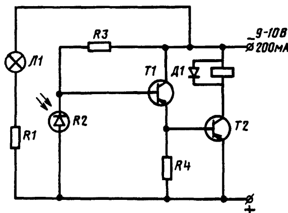
Электрическая схема автоматического датчика
