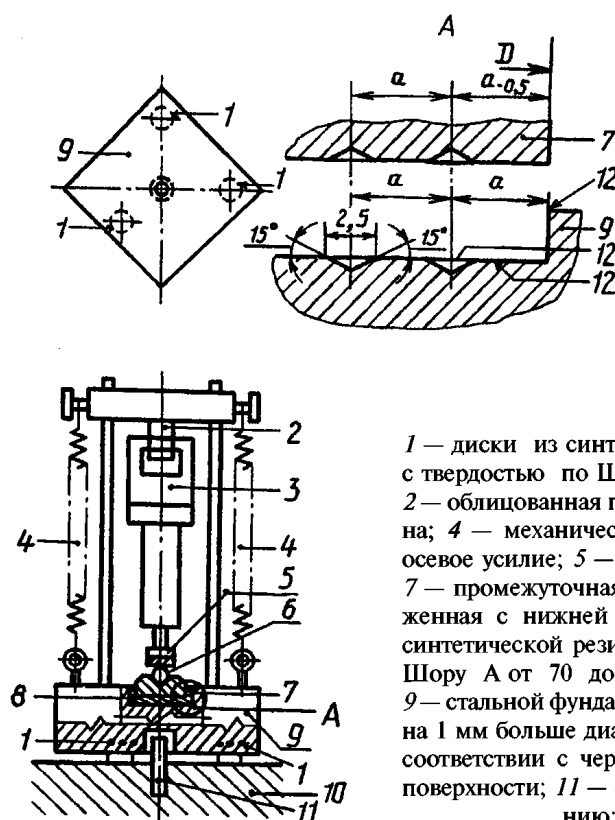
Испытательный прибор
