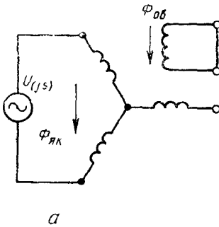
а Продольная ось. Питание двух фаз обмотки якоря
