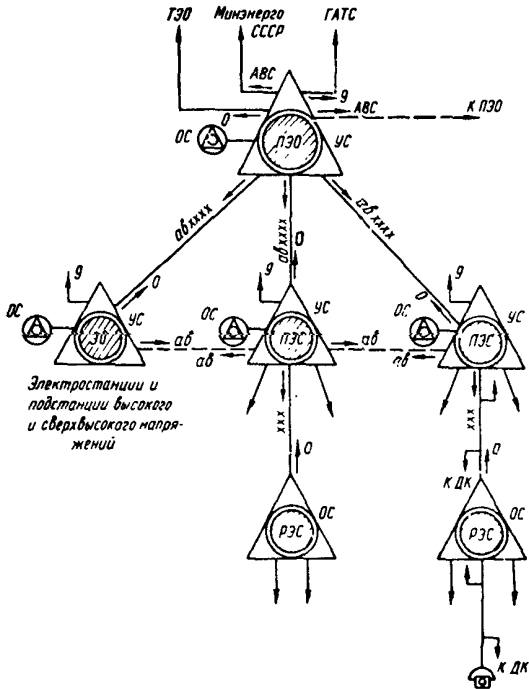
Рис.15. Структурная схема производственно-технологической телефонной сети энергосистемы
