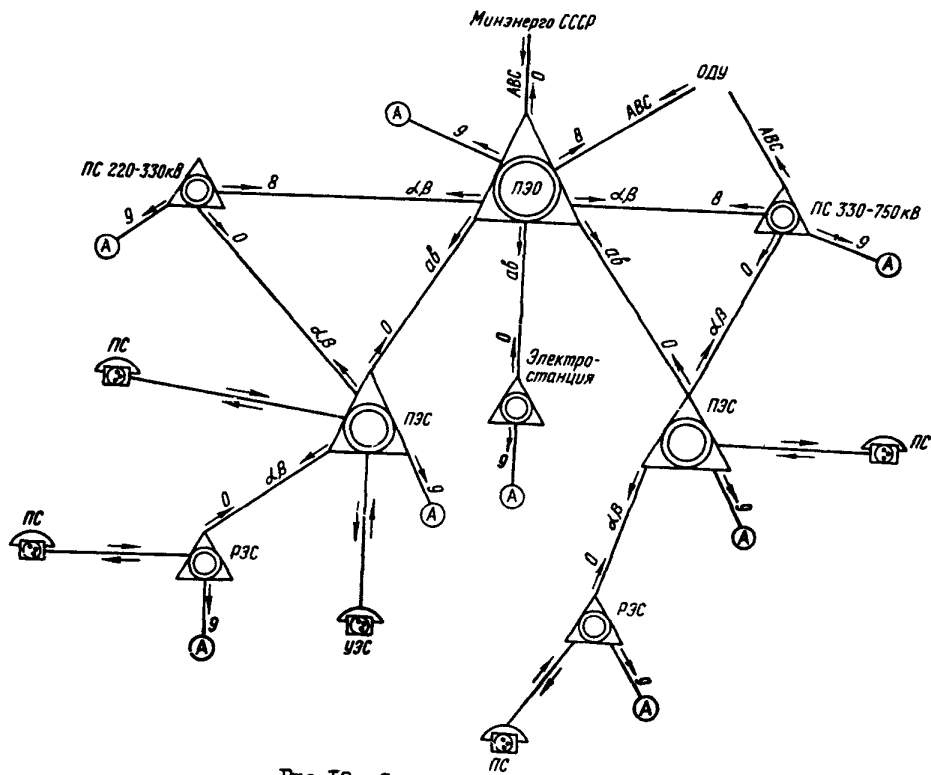
Рис.10. Структурная схема УЭС
