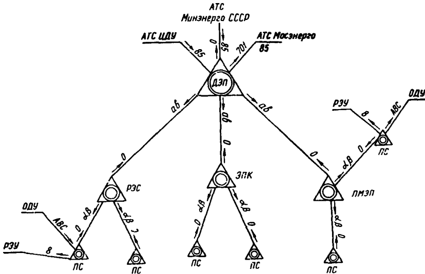
Рис.12. Структурная схема ПТС ДЭП
