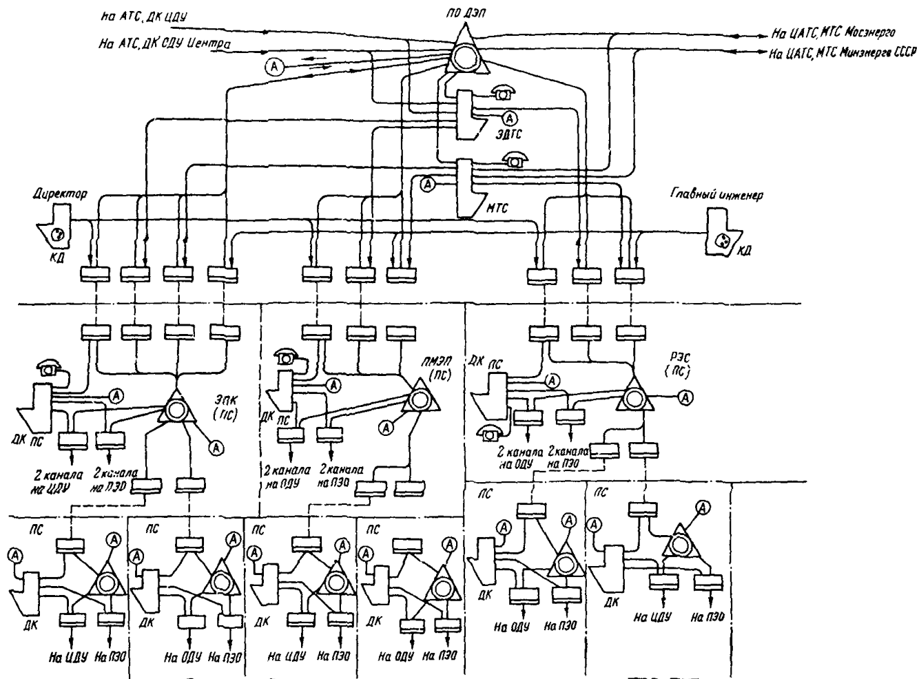
Рис.13. Схема коммутации телефонных каналов МТС ДЭП
