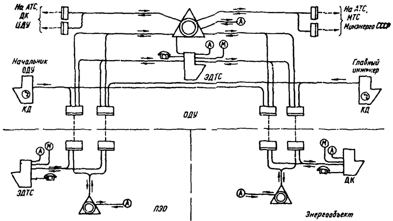
Рис.9. Схема коммутации телефонных каналов ПТС ОДУ
