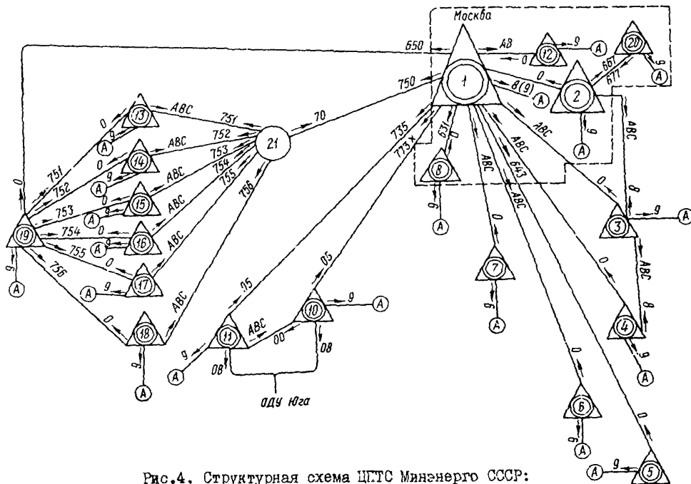
Рис.4. Структурная схема ЦПТС Минэнерго СССР:
