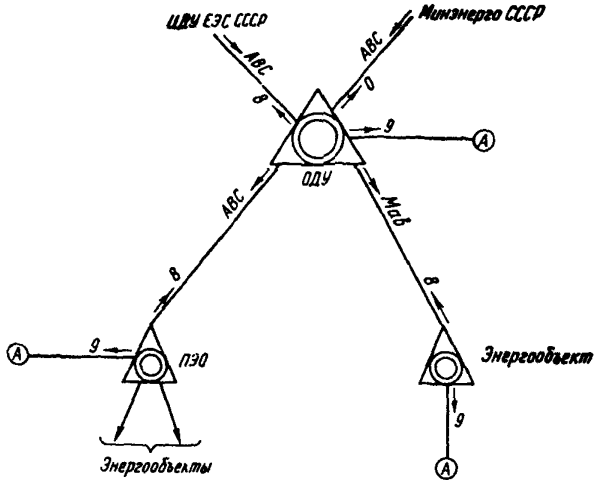
Рис.8. Структурная схема ПТС ОДУ
