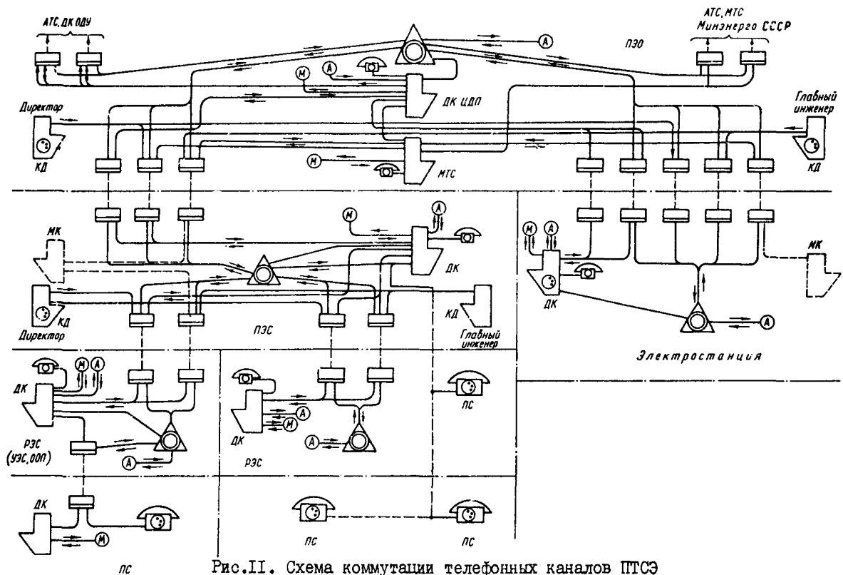
Рис. II. Схема коммутации телефонных каналов РТСЭ
