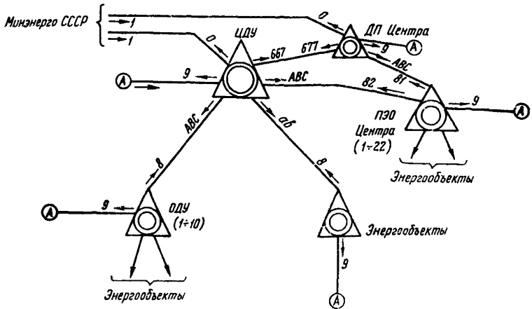
Рис.6. Структурная схема ЦДУ
