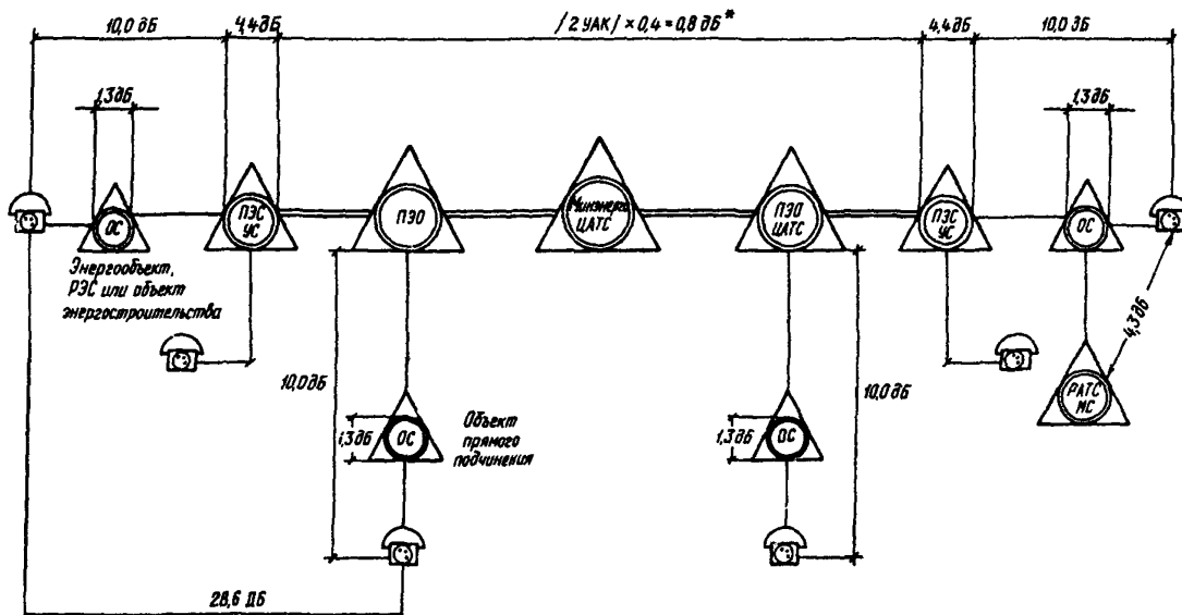
Рис.17. Схема распределения затухания по участкам разговорного тракта
