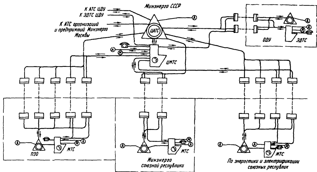
Рис.5. Схема коммутации телефонных каналов ЦПТС Минэнерго СССР
