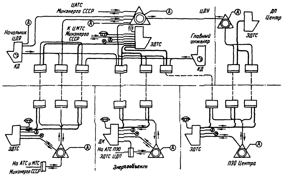
Рис.7. Схема коммутации телефонных каналов ЦАТС ЦДУ
