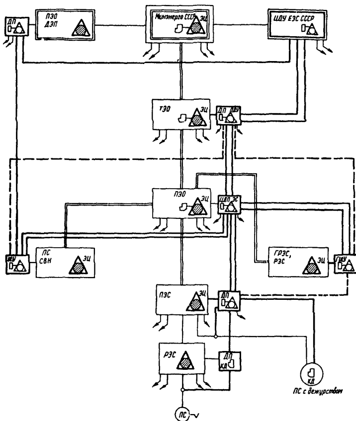
Рис.3. Структурная схема ОДТЭС ЕЭС СССР и ПТЭС Минэнерго СССР на II период (1996-2005 гг.)
