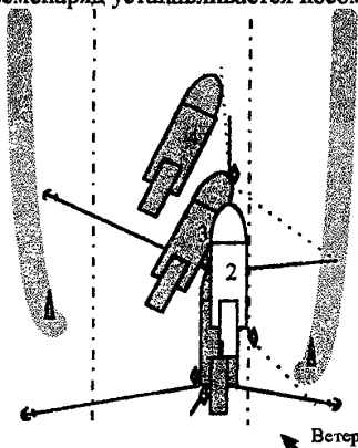
Рисунок 2 Схема съемки земснаряда с участка, расположенного между головками молв 1...4 - положения земснаряда при съемке
