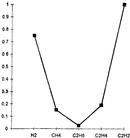
Рис. 4.5. График дефакта электрического характера (дуга), вызванного короткозамкнутым контуром в остане
