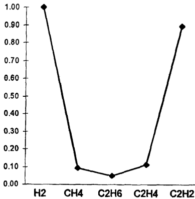
Рис.4.8 График дефекта электрического характера(дуга)
