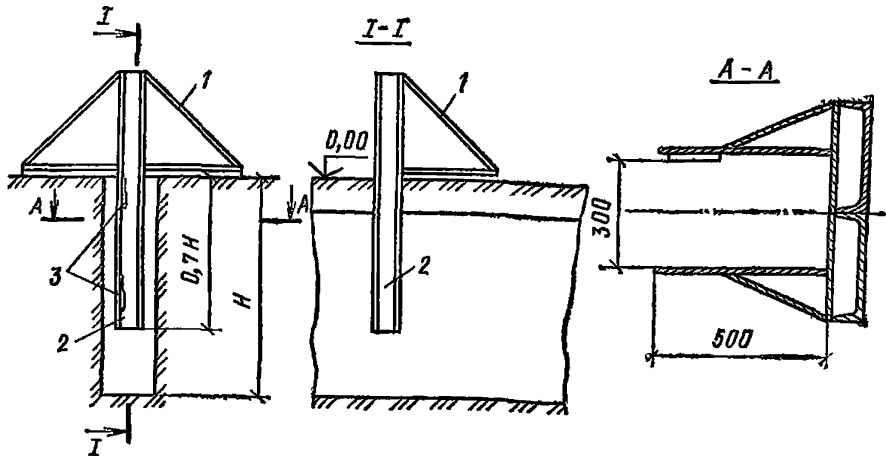
Рис. 83. Кондуктор для монтажа стеновых панелей
