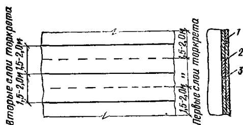
Рис. 92. Порядок нанесения слоев торкрет-гидроизоляции
