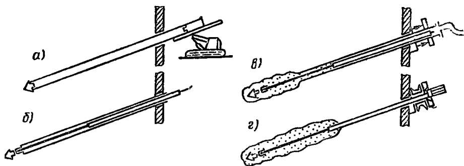
Рис. 1. Технология устройства анкера с тупым башмаком
