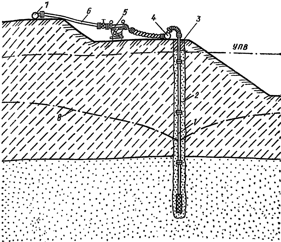
Рис. 48. Схема понижения иглофильтрами в двухслойной среде
