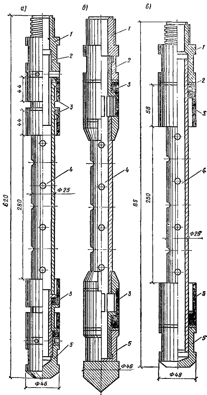
Рис. 63. Конструкция манжетных тампонов
