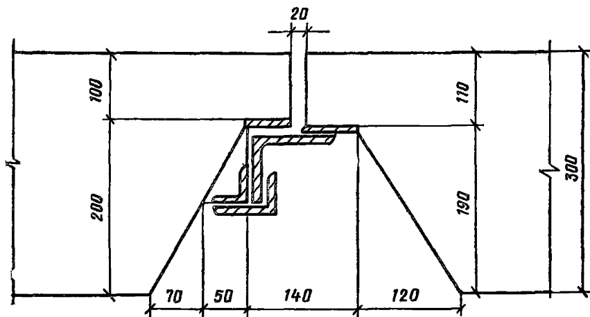
Рис. 86. Стационарная направляющая
