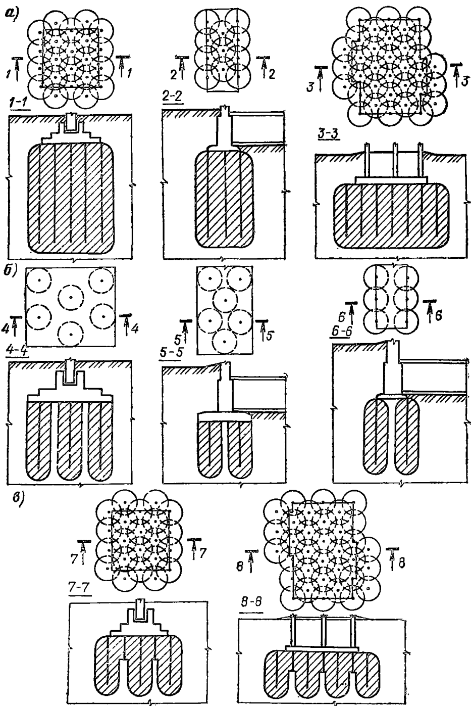
Рис. 55. Конструктивные схемы инъекционного закрепления грунтов а — сплошное закрепление; б — армированное закрепление; в — комбинированное закрепление
