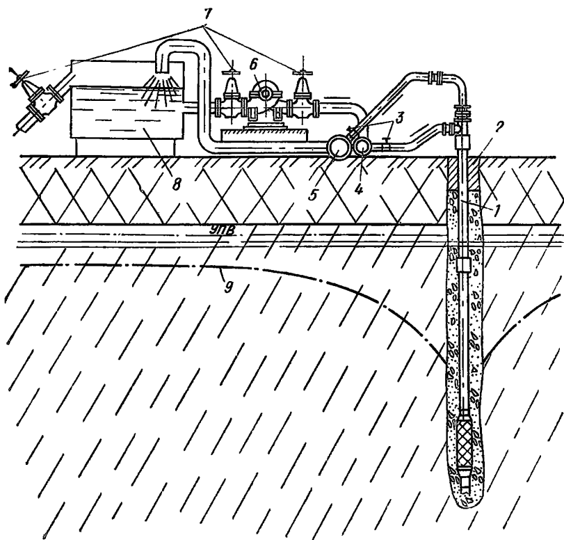
Рис. 50. Установка ЭИ-70 с эжекторными иглофильтрами
