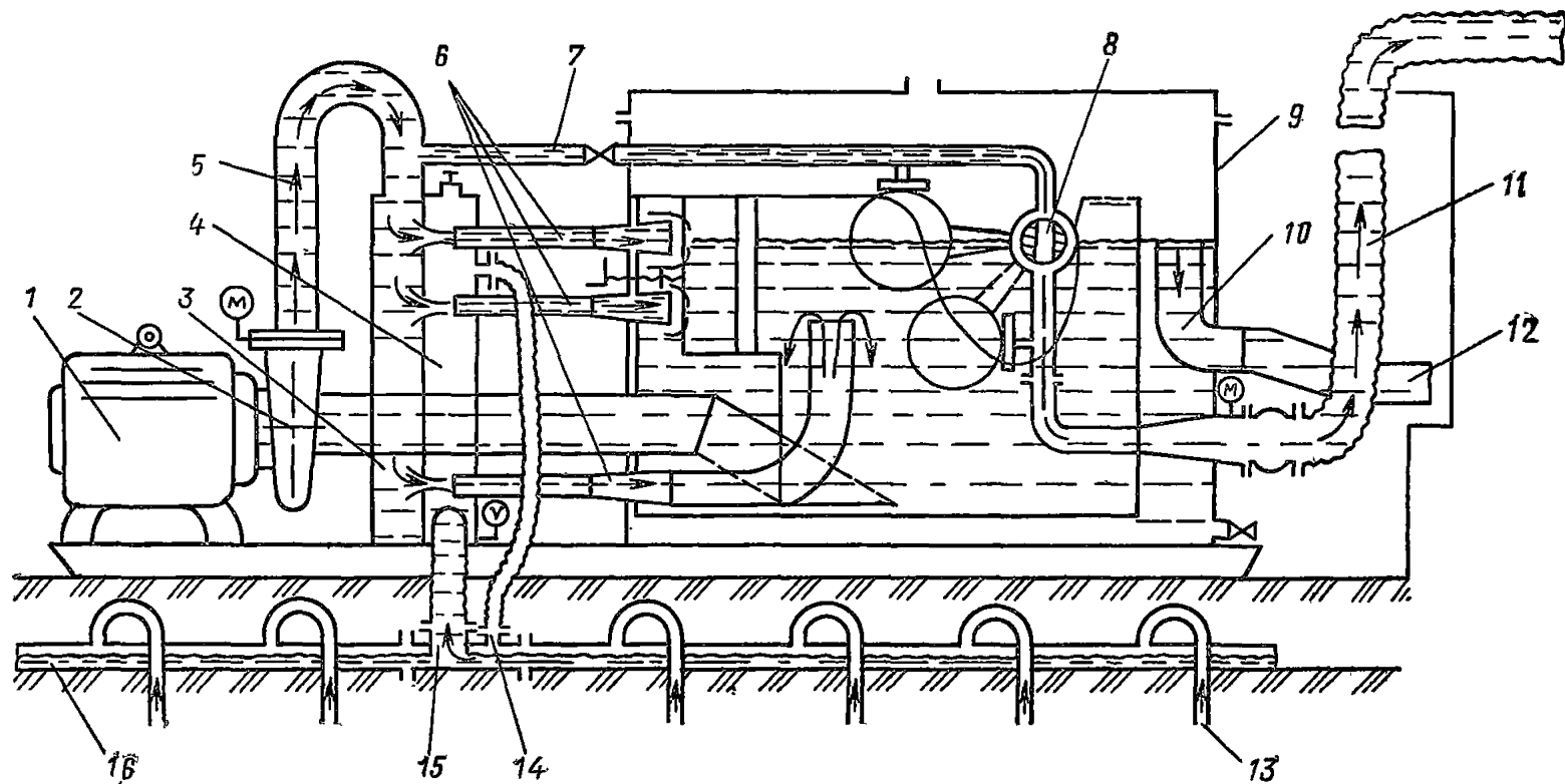
Рис. 49. Схема насосной установки УВВ-3
