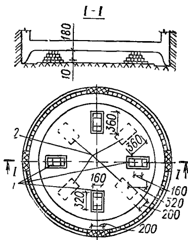
Рис. 111. Последовательность перестановки шпальных клеток
