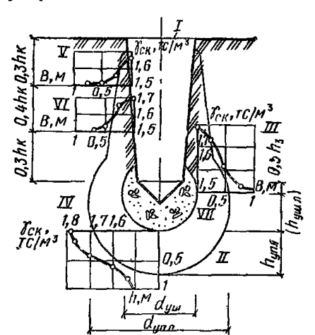
Рис. 17. Уплотненная зона и график изменения объемного веса скелета уплотненных грунтов для удлиненных фундаментов с уширенным основанием
