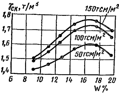
Рис. 14. Графики зависимости удельного веса сухого грунта от влажности при постоянной удельной работе А (А=50, 100, 150 т·см/м)
