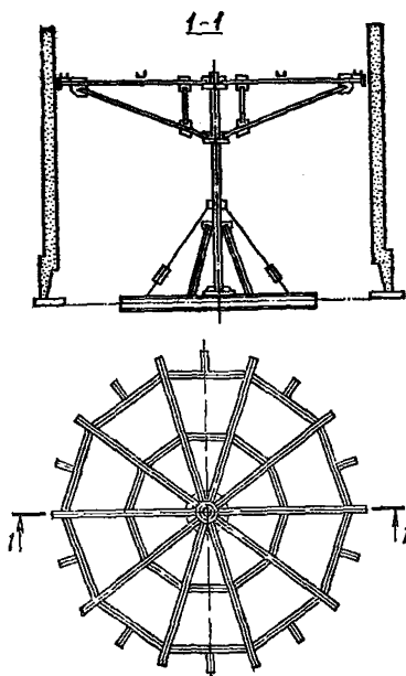
Рис. 98. Кондуктор консольного типа
