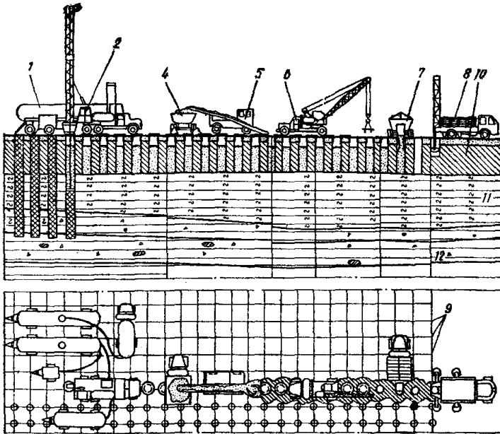
Рис. 2. Укрепление основания бурсмесительным способом с использованием серийной буровой установки с передвижным растворонасосным узлом, с центральной буровой установкой с передвижным растворонасосным узлом, снабженным цементным раствором с центрального бетонорастворного узла
