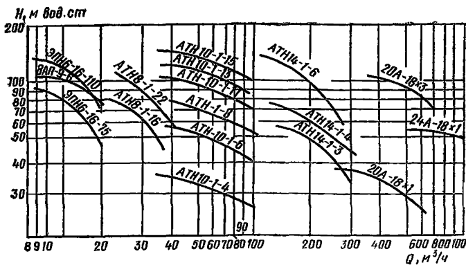
Рис. 30. Характеристики насосов типа А, АП, АТН, ЭПН
