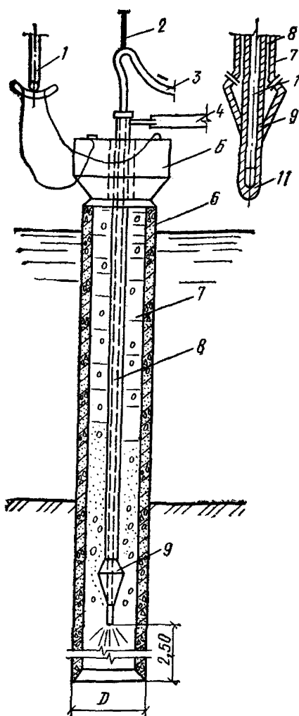
Рис. 1. Схема вибропогружения свая-оболочки с применением пневмоинъектора
