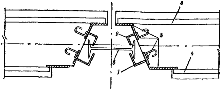
Рис. 84. Съёмная (инвентарная) направляющая
