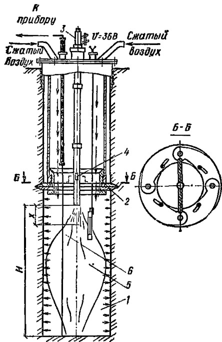
Рис. 74. Схема термического закрепления грунтов с применением многоспальной термопары и винтообразного отсекателя рабочего объема скважины
