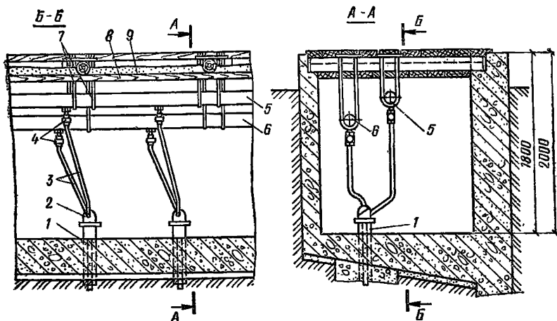
Рис. 77. Расположение рассольных коммуникаций в форшахте
