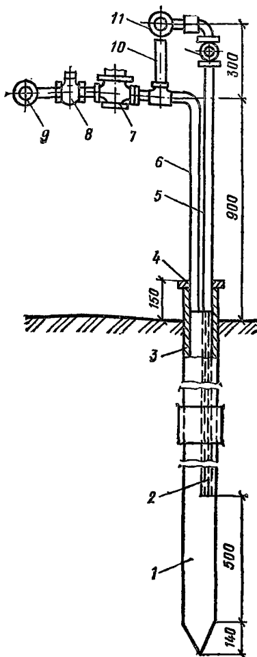
Рис. 78. Замораживающая колонка
