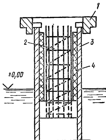
Рис. 6. Схема устройства амортизирующего слоя на сваяе-оболочке
