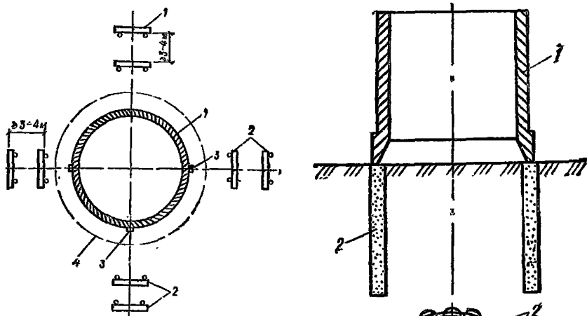
Рис. 89. Схема закрепления основных осей опускаемого колодца или кессона на местности
