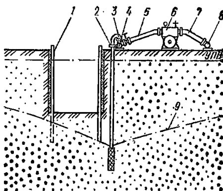
Рис. 43. Линейная система игло-фильтров
