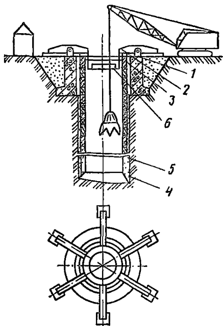
Рис. 107. Технологическая схема погружения колодца способом задавливания
