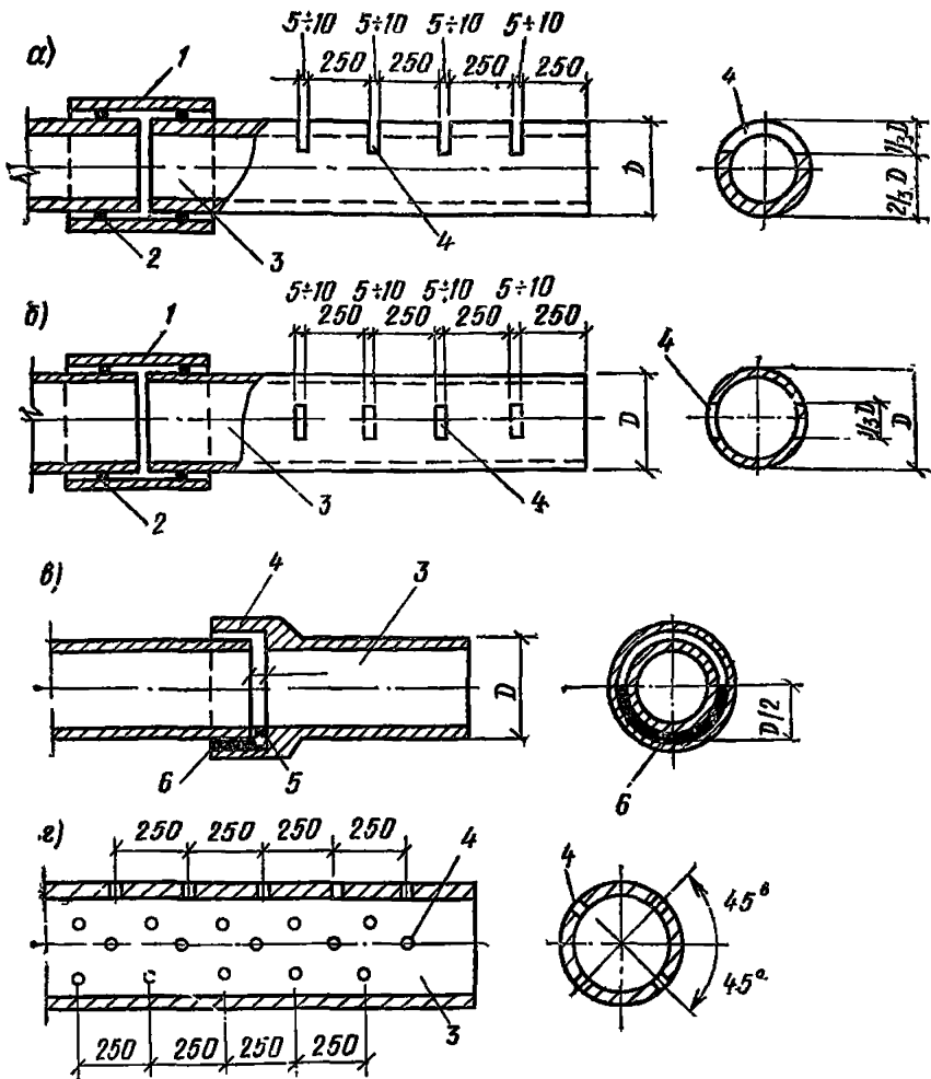
Рис. 28. Водоприемные отверстия в дренажных трубах
