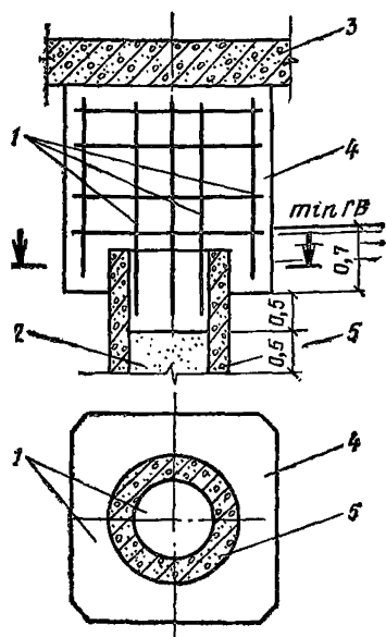
Рис. 4. Свая-оболочка с монолитной железобетонной капителью
