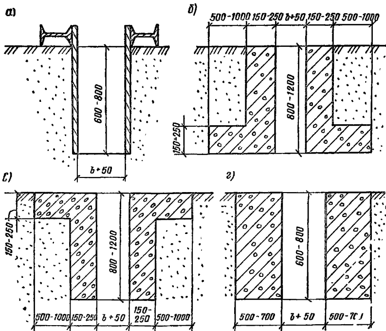
Рис. 80. Конструкции крепления верха траншей
