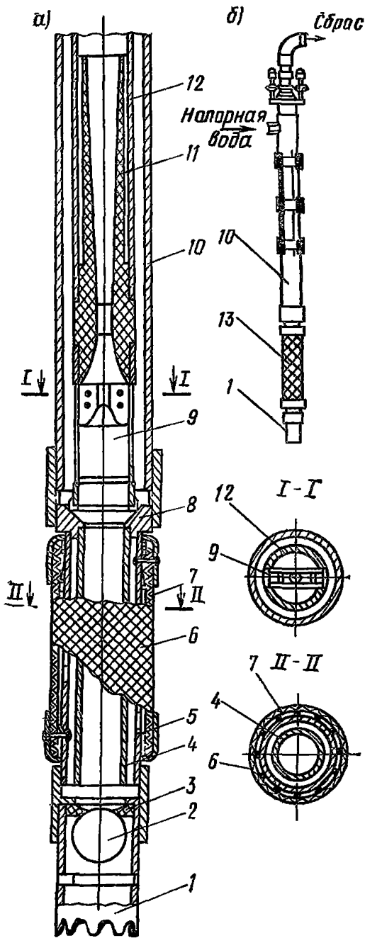
Рис. 51. Эжекторный иглофильтр
