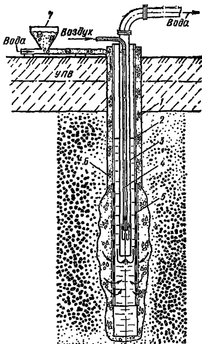
Рис. 42. Схема устройства гидравлическим способом песчано-гравийной обсыпки скважины
