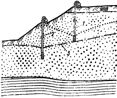
Рис. 45. Схема ярусного водопонижения иглофильтрами
