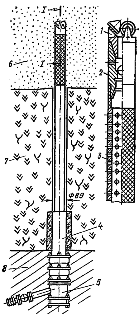
Рис. 37. Восстающая скважина
