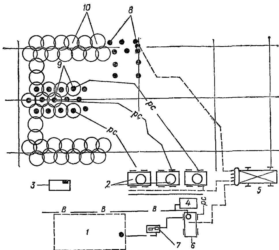
Рис. 56. Схема организации работ по закреплению грунтов через иньекторы 1 — место складирования химреагентов; 2 — пневмоустановки (или насосы), 3 — верстак; 4 — емкость с водой; 5 — компрессор; 6 — емкость для приготовления рабочих растворов; 7 — насос; 8 — погруженные иньекторы; 9 — нагнетание закрепляющих растворов; 10 — закрепленный грунт; В — вода; РС — закрепляющие растворы или смеси
