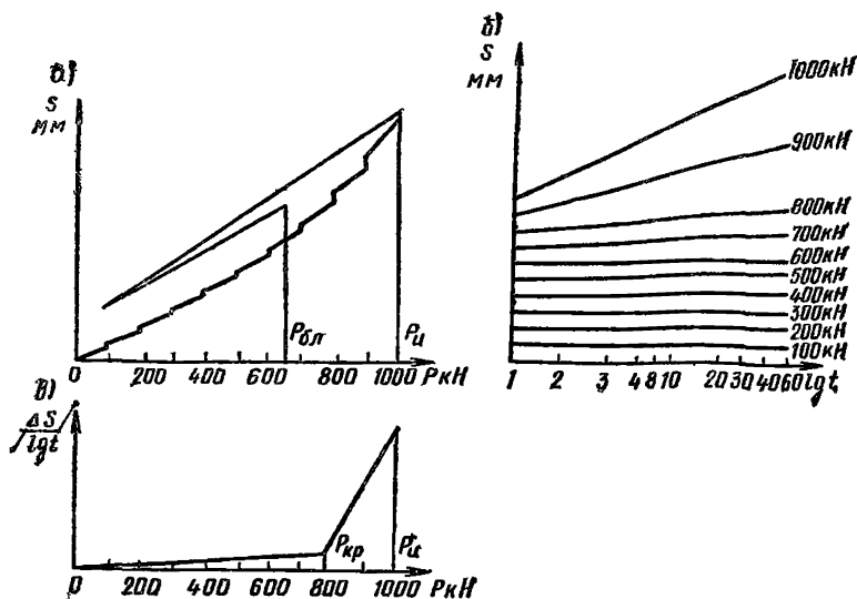
Рис. 1. Контрольные испытания анкеров
