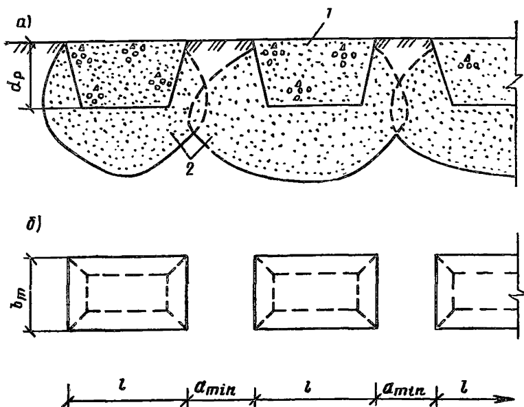
Рис. 2. Ленточные прерывистые фундаменты в вытрамбованных котлованах a — разрез по ленточным прерывистым фундаментам; б — вид в плане; 1 — ленточный прерывистый фундамент; 2 — уплотненная зона
