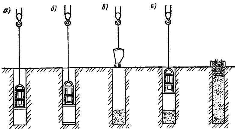
Рис. 1. Изготовление набивных свай с помощью виброгрейферов
