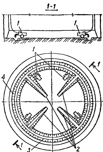
Рис. 102. Схема открытого водоотлива
