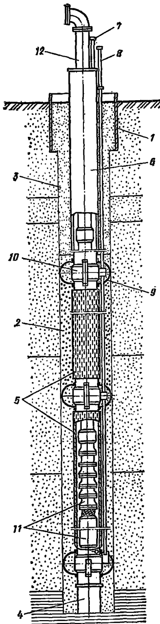
Рис. 33 Открытая скважина, оборудованная насосом
