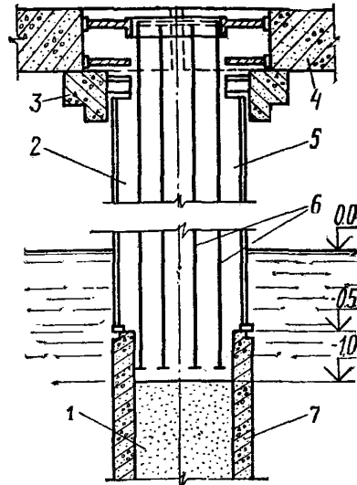
Рис. 3. Свая-оболочка со стальным верхним звеном, бетонируемым «всухо»
