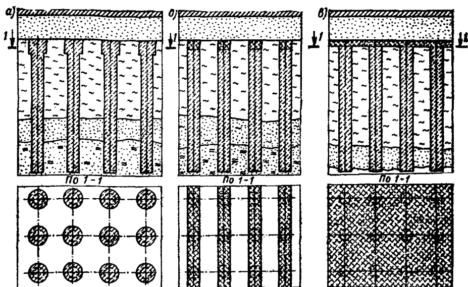
Рис. 72. Схемы устройства оголовков илоцементных свай в виде а — капителей; б — балок; в — плиты
