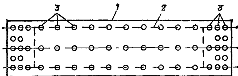
Рис. 25. Рекомендуемая схема расположения скважин для замачивания котлованов
