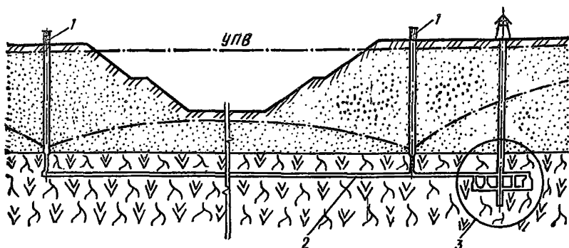
Рис. 39. Система водопонижения со сквозными фильтрами
