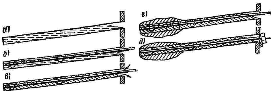
Рис. 3. Технология устройства анкера с инъекционной трубкой
