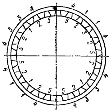
Рис. 94. Последовательность снятия колодцев с деревянных подкладок
