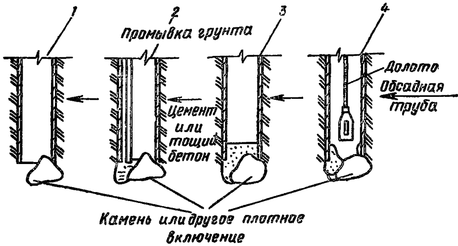
Рис. 6. Рекомендуемые мероприятия по предупреждению искривлений скважин
