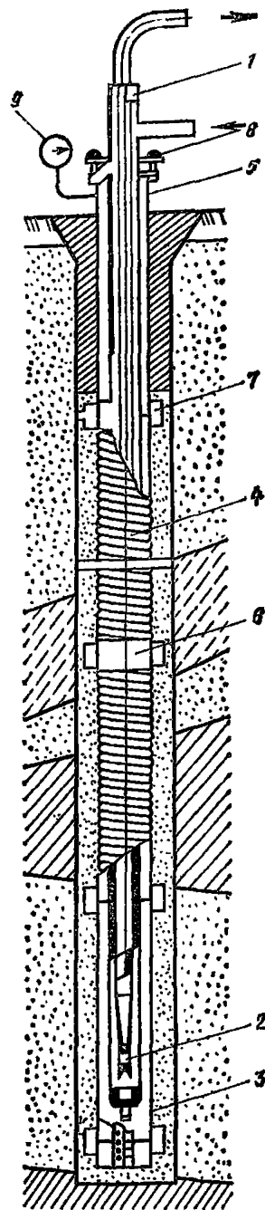
Рис. 52. Вакуумная концентрическая сыважина
