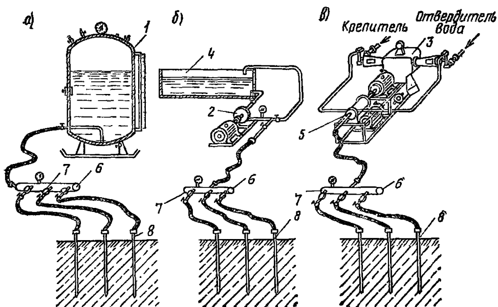
Рис. 67. Технологические схемы нагнетания закрепляющих растворов в грунты а — с использованием пневмобака; б — насоса; в — дозирочного агрегата; 1 — пневмобак; 2 — насос; 3 — дозирочный агрегат; 4 — емкость с раствором; 5 — смеситель; 6 — распределитель; 7 — счетчики расхода; 8 — инъекторы
