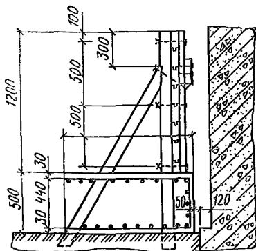
Рис. 100. Конструкция ограждения форшахты
