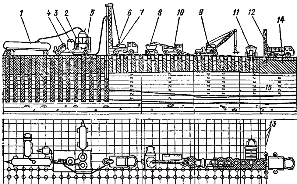
Рис. 3. Укрепление основания буромесительным способом с использованием серийной установки, с передвижным растворомасосным узлом, снабженным готовым цементным раствором с центрального бетонорастворного узла
