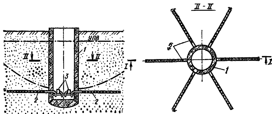
Рис. 36. Лучевой водозабор
