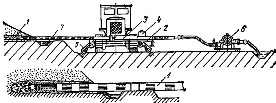
Рис. 35. Схема устройства горизонтальной скважины
