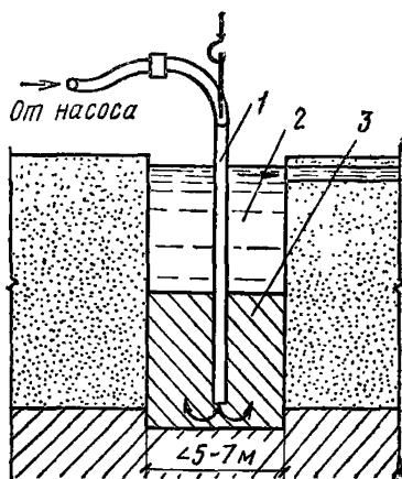
Рис. 87. Схема заполнения секции траншеи глиноцементным раствором
