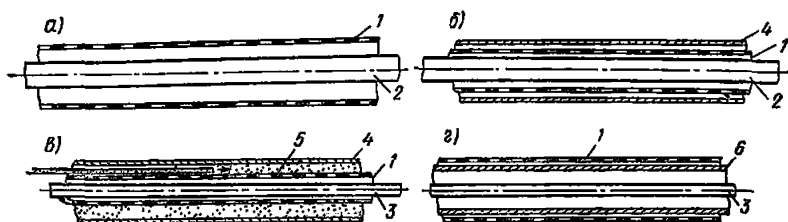
Рис. 41. Схемы устройства горизонтальных скважин
