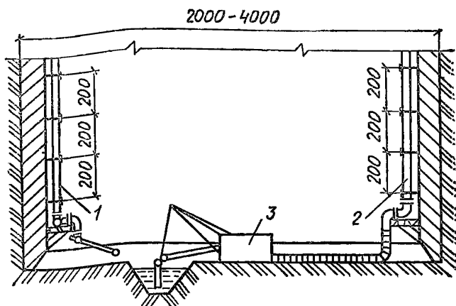
Рис. 105. Разработка грунта землесосом 1 — водовод; 2 — пульповод; 3 — землесос
