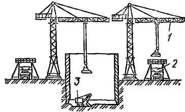
Рис. 104. Разработка грунта экскаватором 1 — башенный кран; 2 — бункер; 3 — экскаватор
