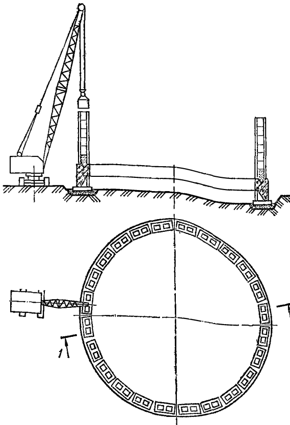
Рис. 96. Монтаж сборно-монолитного колодца из пустотных блоков
