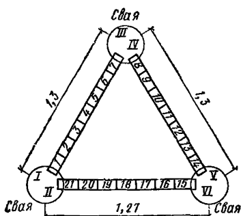
Рис. 18. Схема отбора образцов грунта для определения плотности грунта
