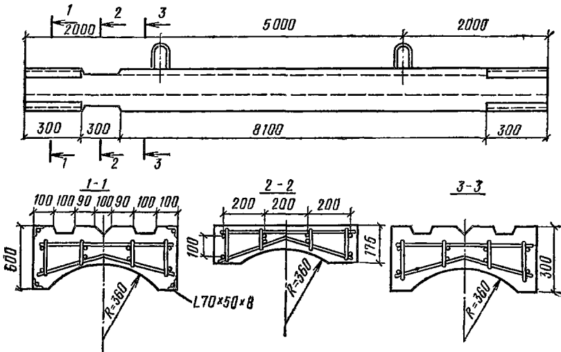
Рис. 82. Неизвлекаемый железобетонный ограничитель
