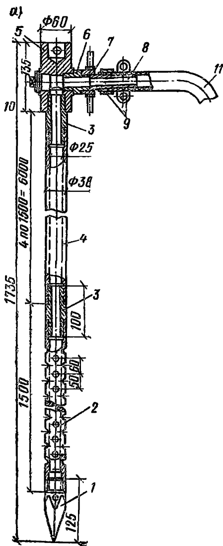
Рис. 58. Конструкция забивного инъ-ектора для силикатизации и смолизации песчаных грунтов
