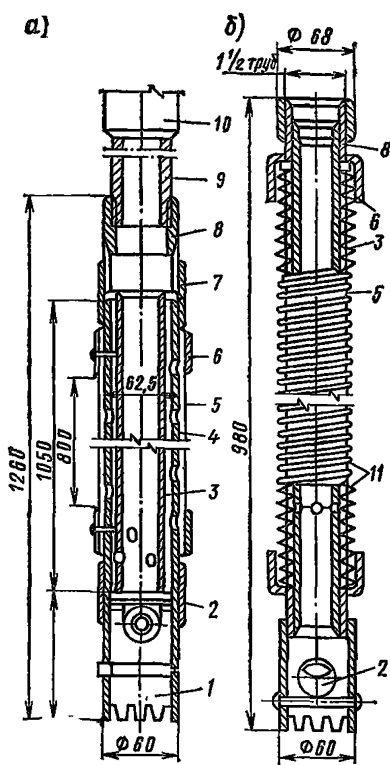
Рис. 48. Конструкция иглофильтров
