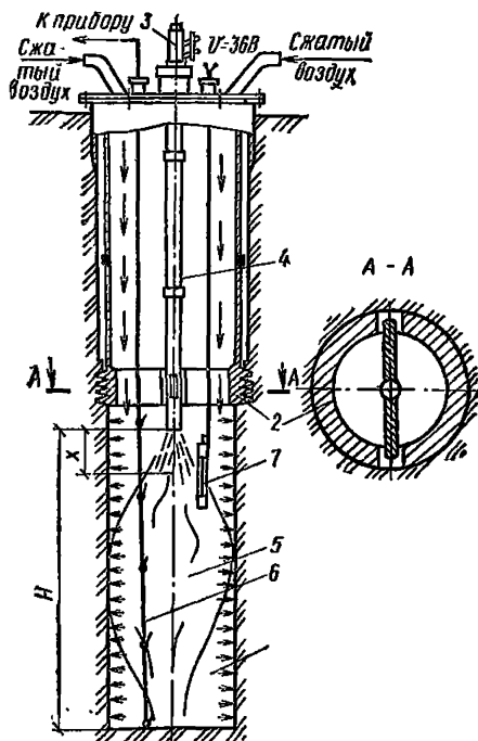
Рис. 75. Схема термического закрепления грунтов с применением термопары передвигного действия и отсекателя рабочего объема скважины с раздвижными ножами
