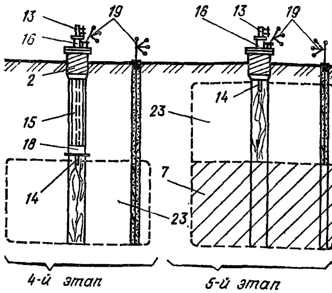
Рис. 3. Технологическая схема выполнения основных этапов 4—5
