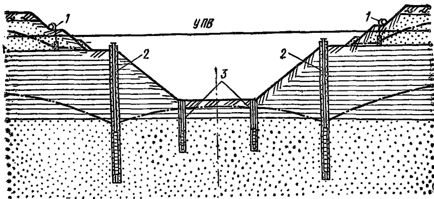
Рис. 34. Система водопонижения с применением резервных самоизливающихся скважин
