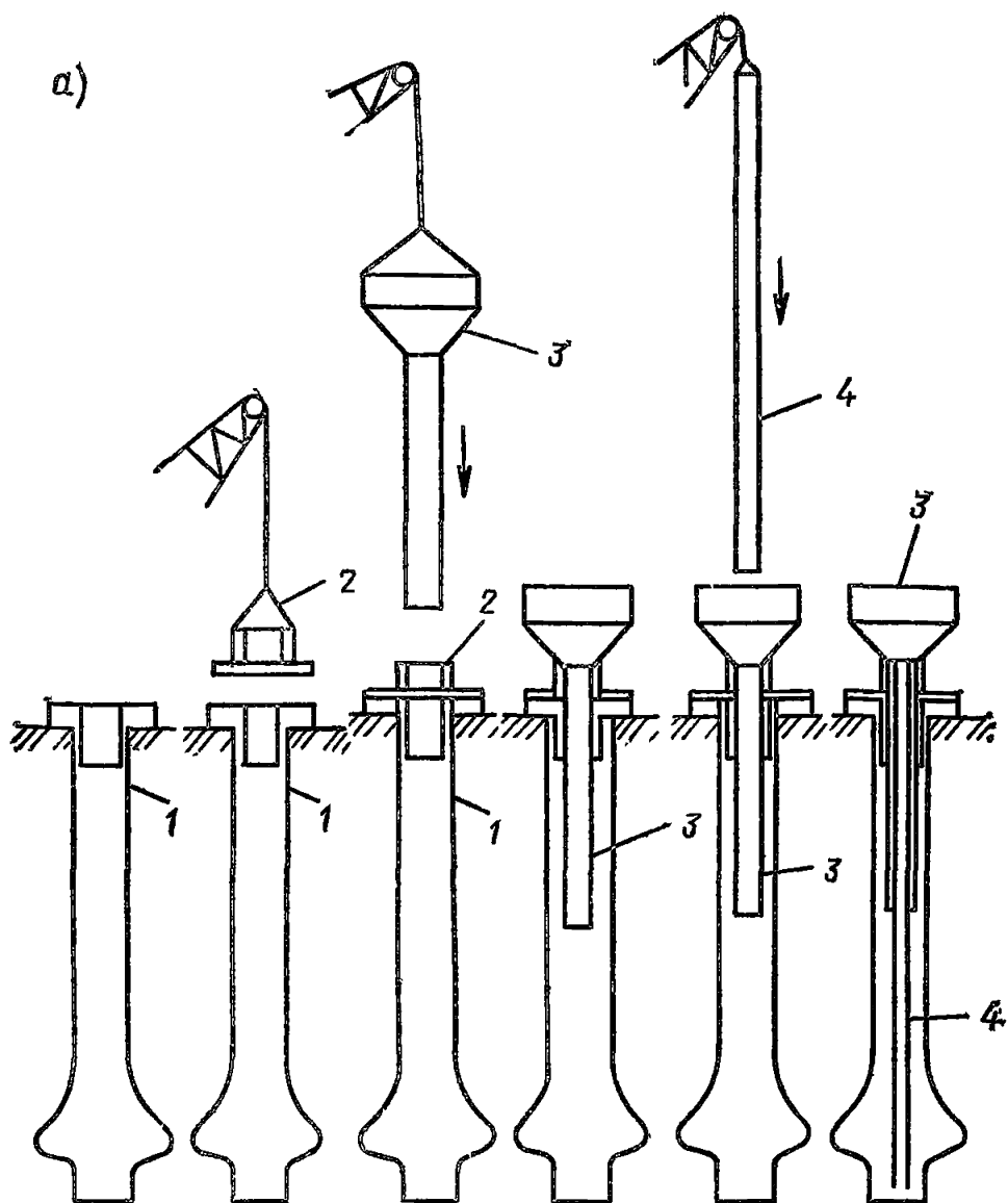
Рис. 8. Бетонирование скважин для свай методом ВПТ
