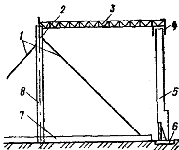
Рис. 98. Кондуктор консольного типа
