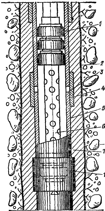
Рис. 62. Схема манжетно-тампонного иньектора
