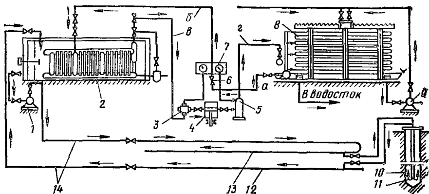
Рис. 76. Схема работы замораживающей станции
