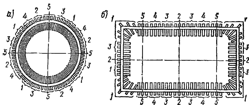
Рис. 94. Последовательность снятия колодцев с деревянных подкладок
