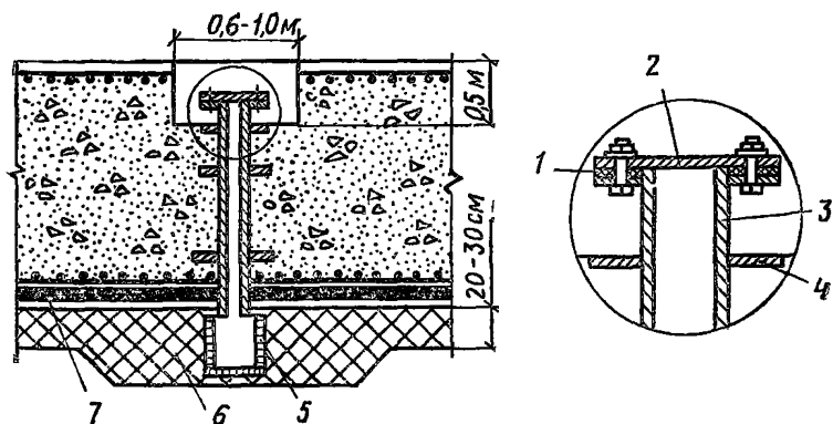
Рис. 106. Устройство для откачки грунтовых вод из-под дна
