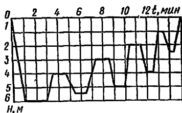
Рис. 27. Технологический график уплотнения песчаного грунта
