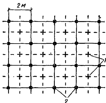
Рис. 26. Схема расположения точек рыхания и уплотнения
