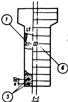
Рис 3 Схема зарисовки трещин на опорном участке балки 16В-18-3 серии ПК-01-06 1-околы бетона, 2-стержни \phi 6 мм, 3-нагретые проволки; 4-клиновидный маяк, 5-разрыв маяка по трещине; 6-участок балки недоступный для осмотра. Цифры у трещин обозначают величину их раскрытия в мм.
