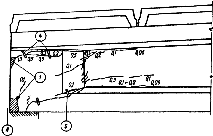
Рис 3 Схема зарисовки трещин на опорном участке балки 16В-18-3 серии ПК-01-06 1-околы бетона, 2-стержни \phi 6 мм, 3-нагретые проволки; 4-клиновидный маяк, 5-разрыв маяка по трещине; 6-участок балки недоступный для осмотра. Цифры у трещин обозначают величину их раскрытия в мм.
