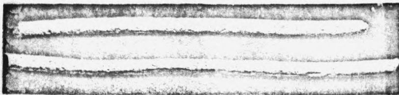
Рис.9. Язвенная коррозия арматуры ригеля перекрытия здания химводоочистки.
