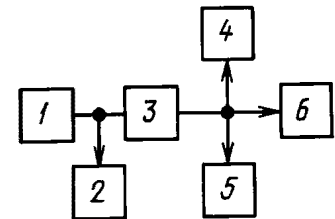
1 — генератор; 2 и 5 — электронный вольтметр; 3 — усилитель мощности; 4 — измеритель коэффициента гармоник; 6 — эквивалент нагрузки усилителя мощности
