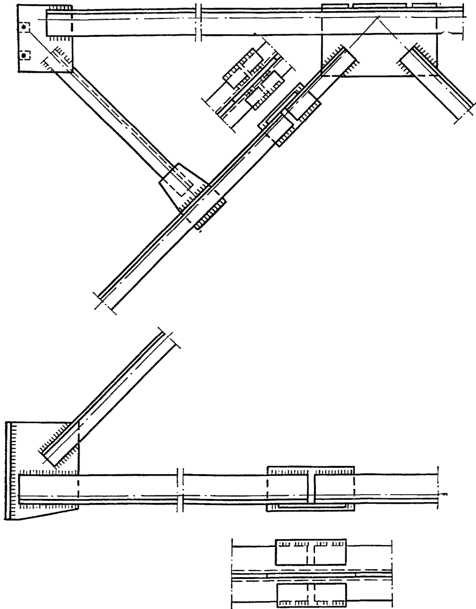
Рис. 54. Пример усиления фермы заменой поврежденных раскосов и участка пояса или выправлением погнутого элемента (жирными линиями показаны новые элементы)
