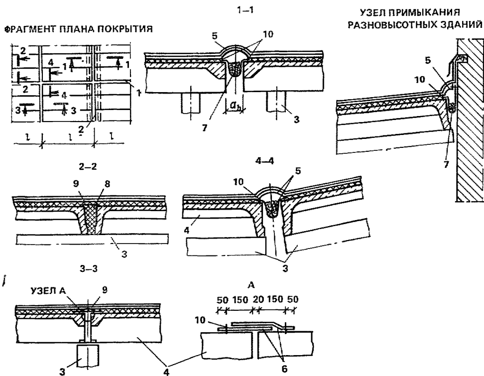
Рис. 36. Устройство узлов в покрытии и кровле
