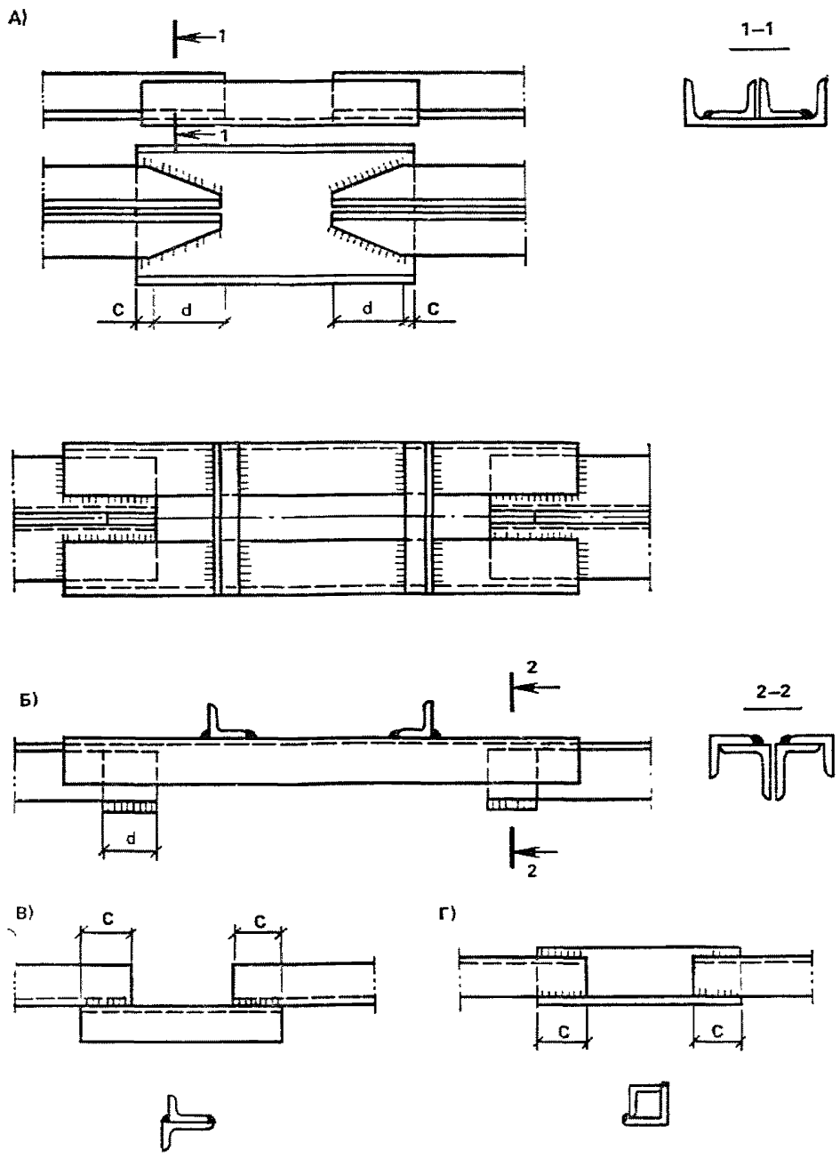
Рис. 50. Восстановление элементов ферм вырезанием и заменой поврежденной части А, Б — элементов из парных уголков; В, Г — элементов из одиночного уголка
