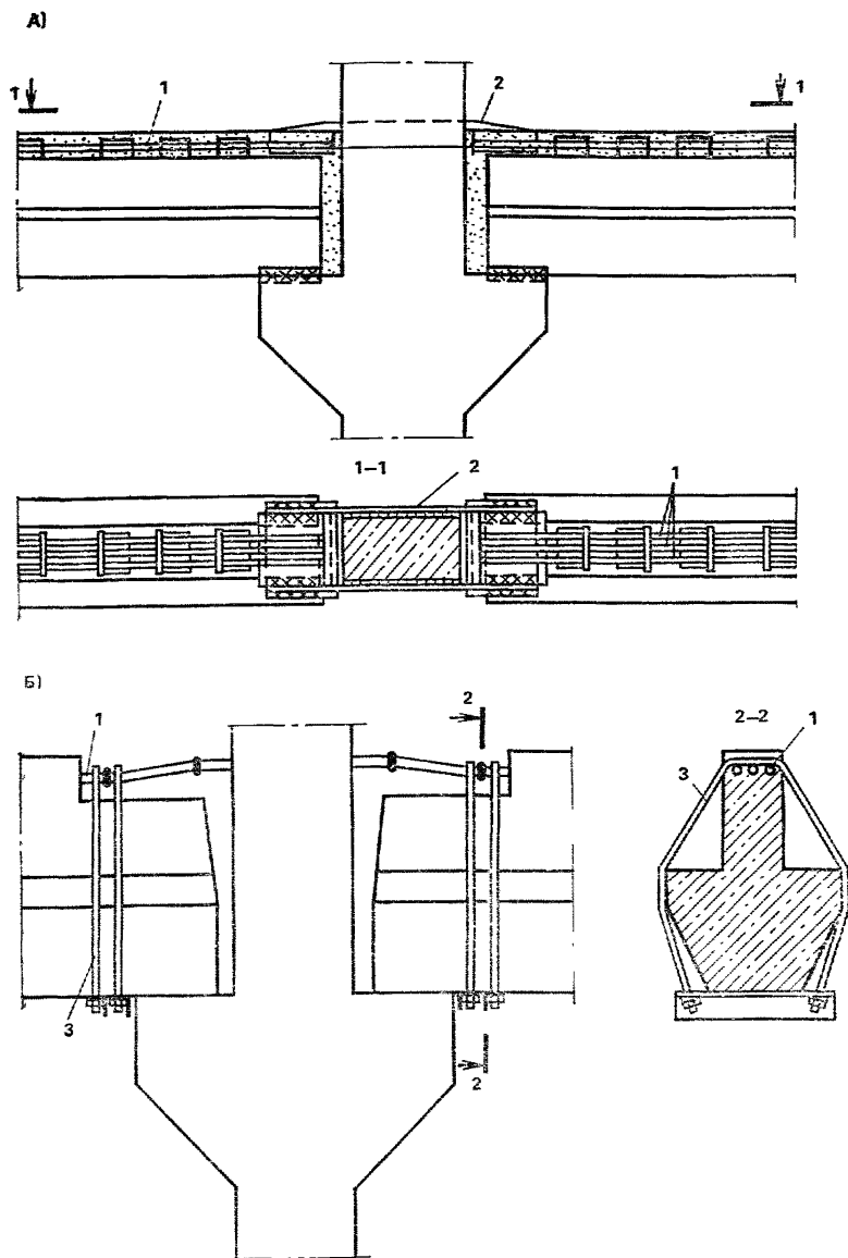
Рис. 34. Усиление узлов сопряжений ригелей с колоннами каркасов многоэтажных производственных зданий при разрыве или искривлении надопорных стержней
