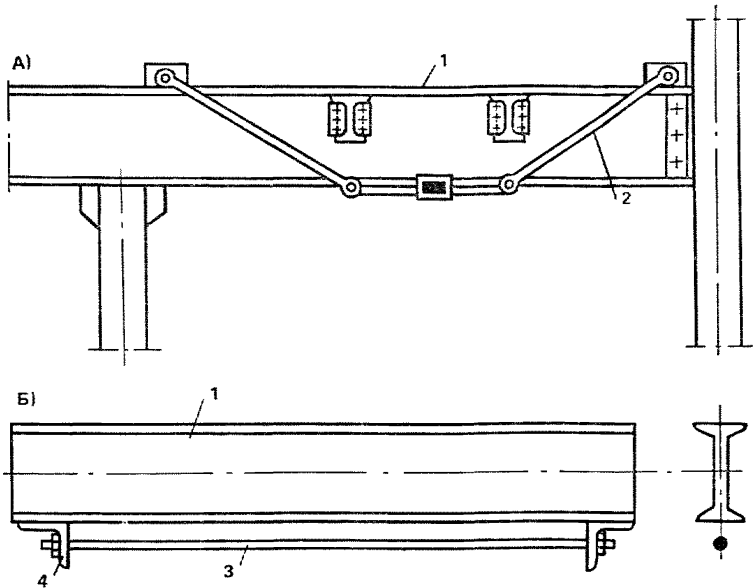
Рис. 42. Примеры усиления балок
