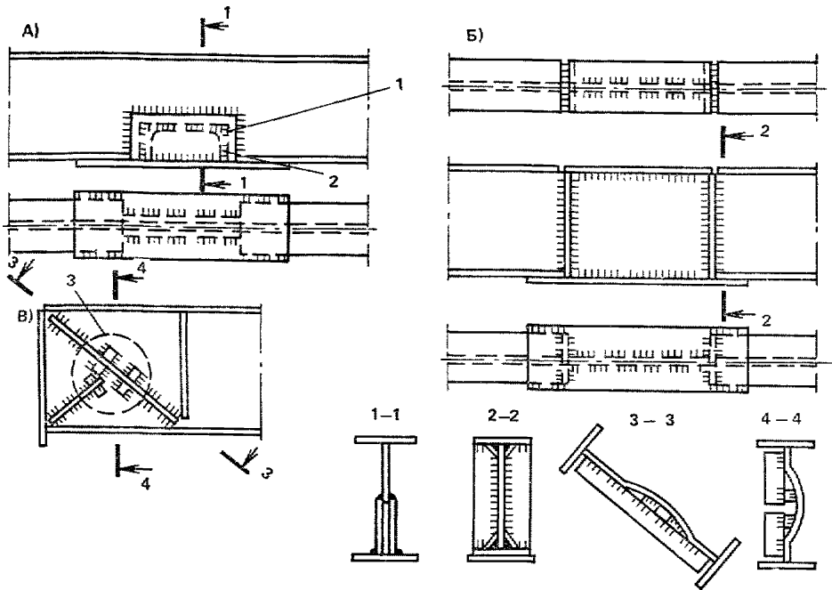
Рис. 41. Исправление повреждений сварных балок
