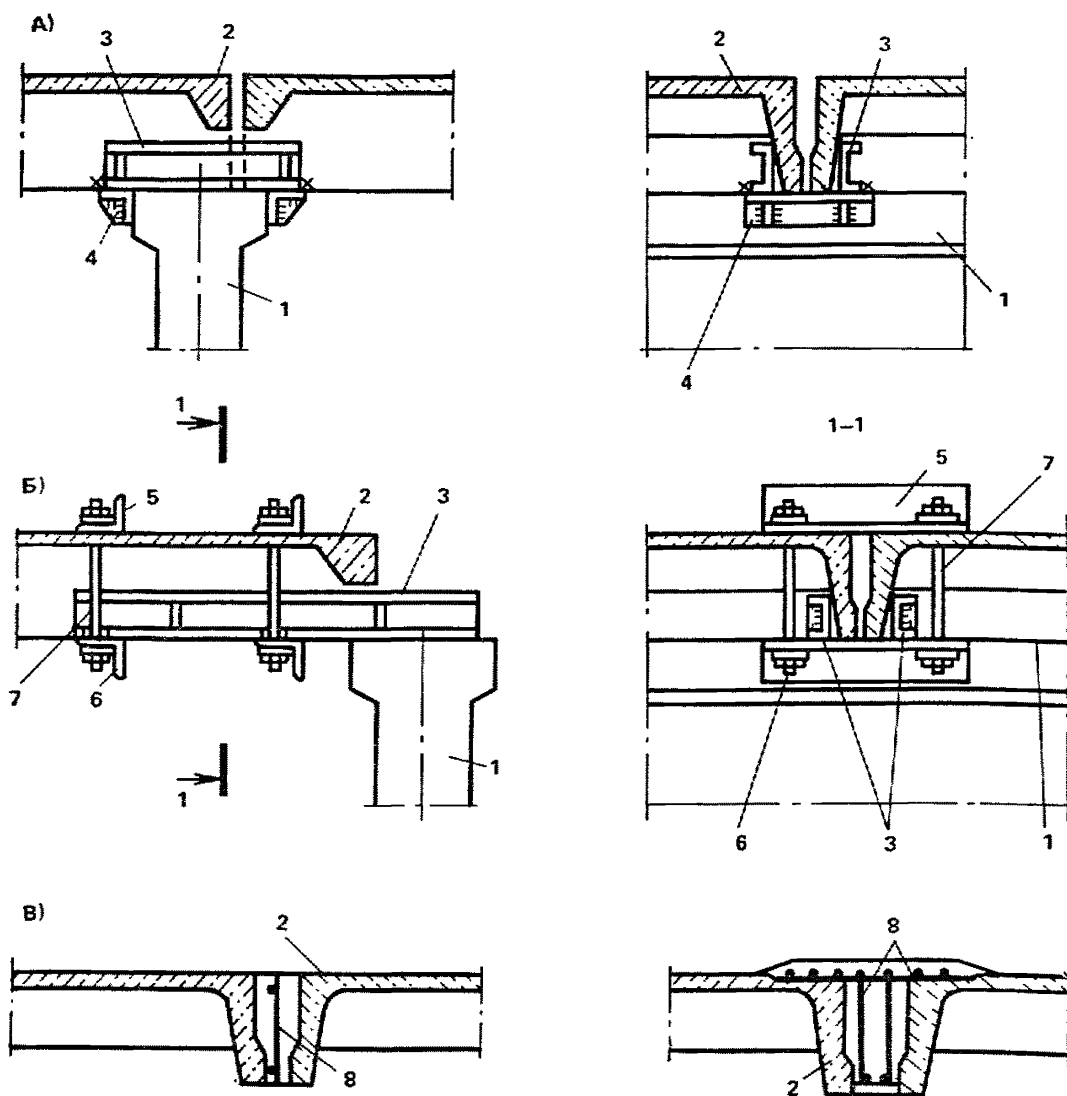
Рис. 6. Усиление опирания при сдвиге плит
