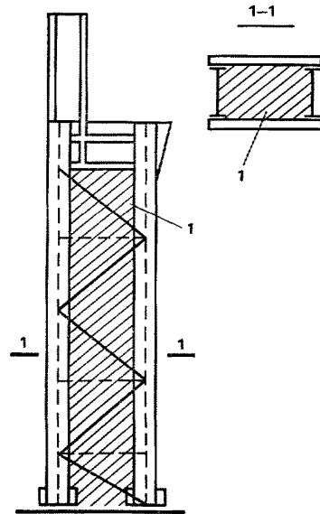
Рис. 64. Усиление колонн бетонированием при искривлении ветвей (1 — бетон)
