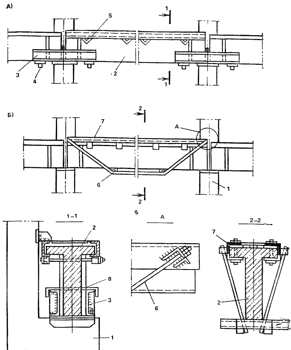
Рис. 18. Усиление подкрановых балок
