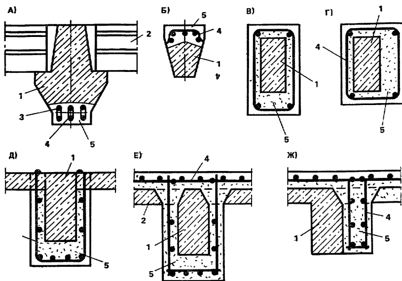
Рис. 11. Схемы сечений балок, усиленных железобетоном
