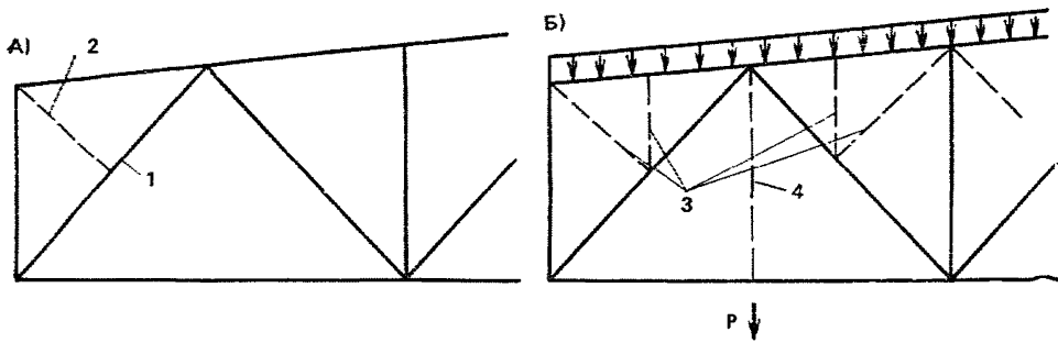
Рис. 43. Усиление фермы
