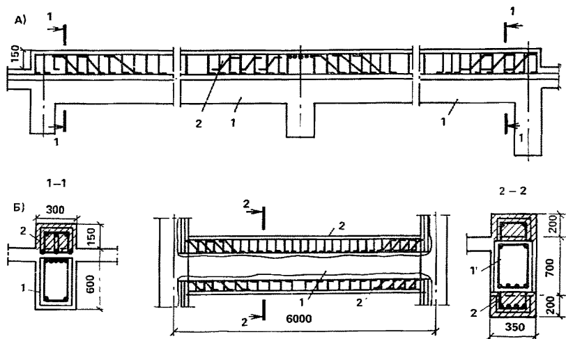
Рис. 15. Усиление балок перекрытий наращиванием
