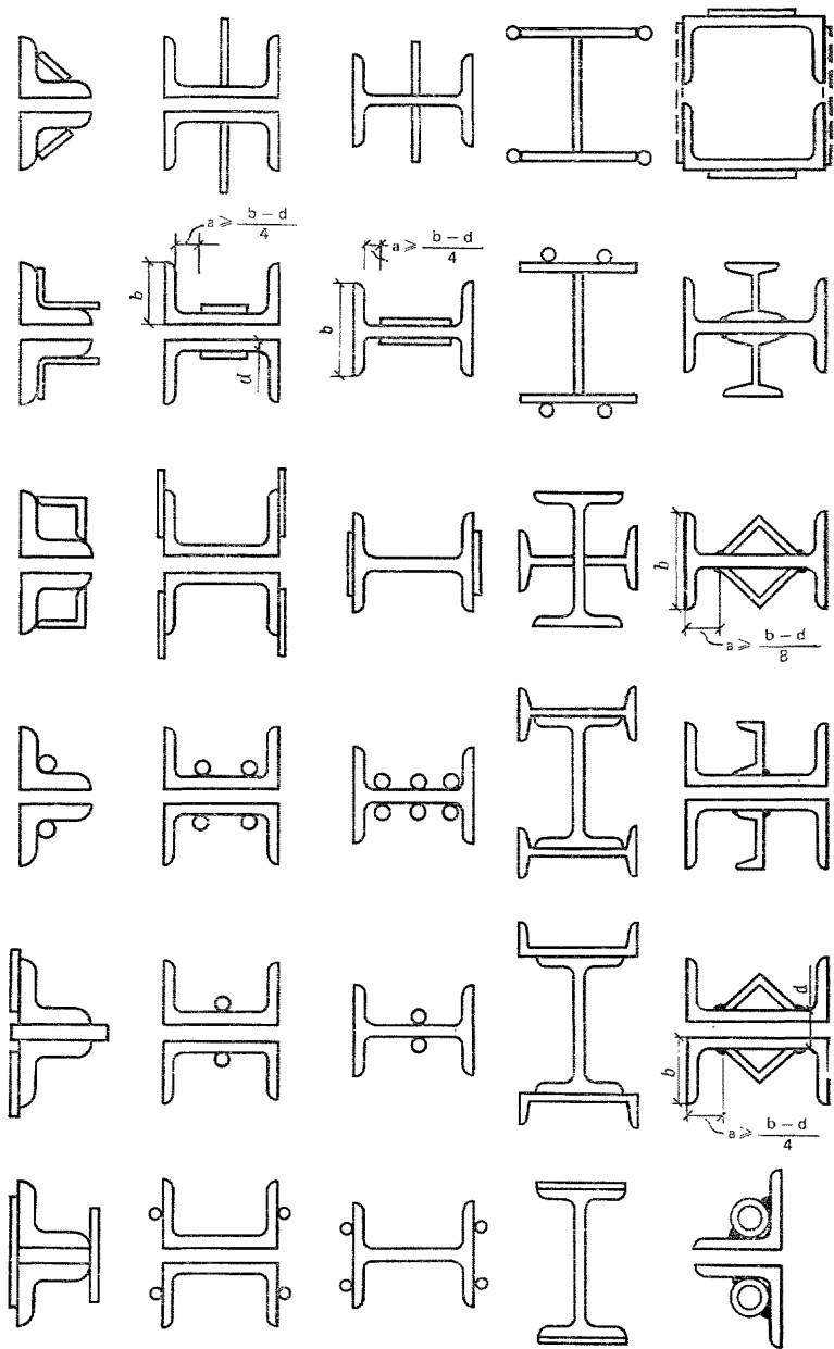
Рис. 49. Усиление сечений центрально-растянутых и центрально-сжатых элементов
