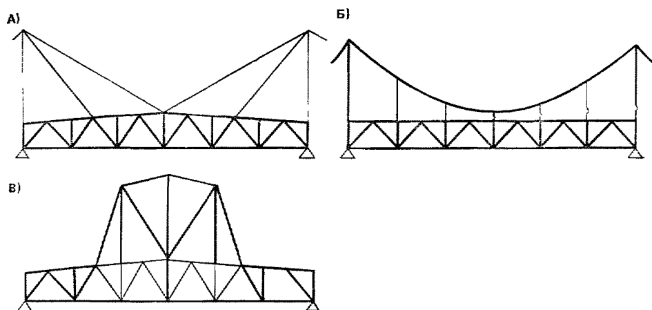
Рис. 45. Схемы усиления ферм
