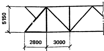
Рис. 54. Пример усиления фермы заменой поврежденных раскосов и участка пояса или выправлением погнутого элемента (жирными линиями показаны новые элементы)
