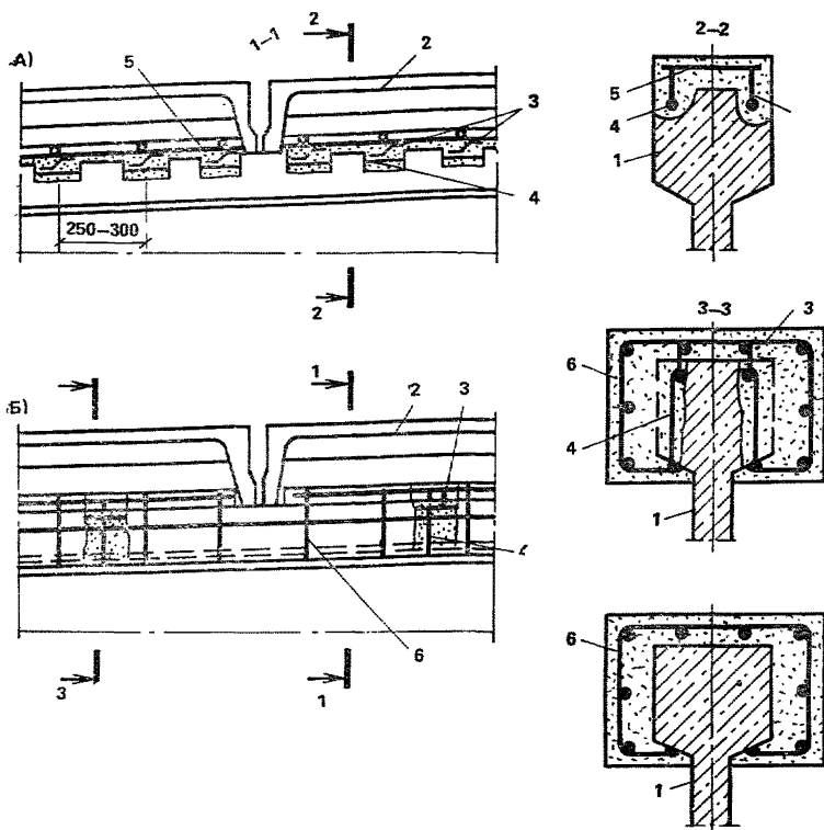
Рис. 13. Усиление сжатого пояса балок
