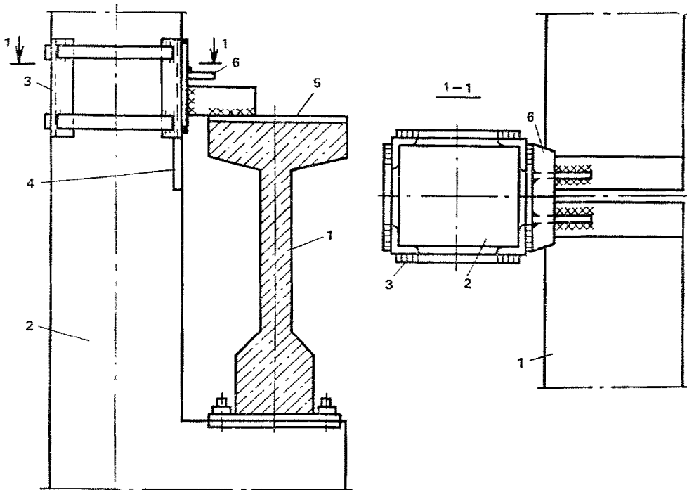
Рис. 20. Усиление (восстановление) крепления подкрановых балок к колонне с приваркой к обойме (сжиму) на сжатой полке 1 — балка; 2 — колонна; 3 — обойма колонны; 4 — закладная деталь; 5 — торцевой лист; 6 — ребро жесткости лицевого листа обоймы на колонне
