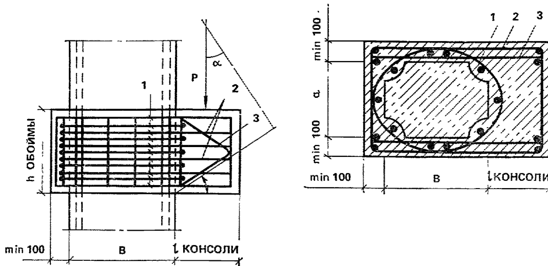
Рис. 26. Осуществление новых консолей (упоров) с устройством обоймы на стволе колонны 1 — спираль обоймы; 2 — хомуты; 3 — отгибы
