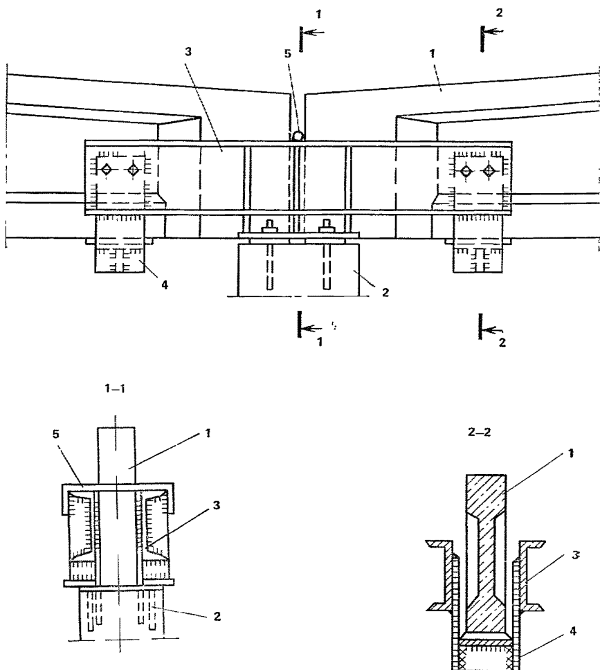
Рис. 17. Усиление балок выносными опорами
