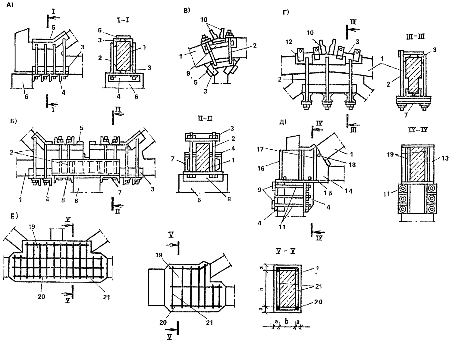
Рис 31. Усиление опорных и промежуточных узлов
