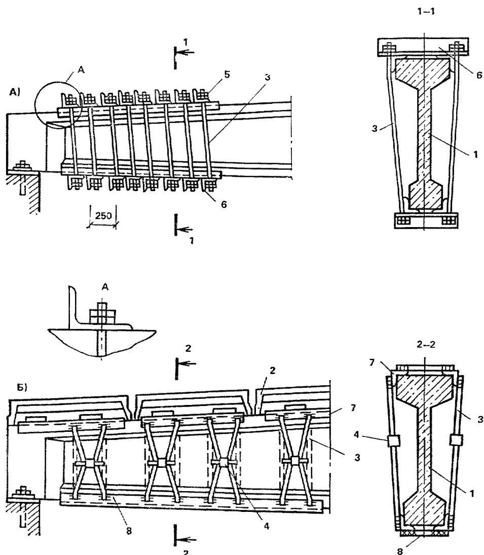
Рис. 14. Усиление опорных участков балок хомутами
