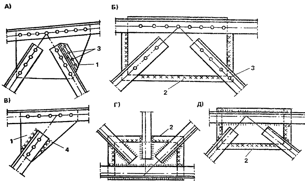
Рис. 48. Усиление фермы дополнительными коротышами и косынками А — постановкой коротышей на заклепках; увеличением размеров в клепа-ных (Б) и сварных (Г, Д) фермах; В — обваркой существующего заклепоч-ного соединения; 1 — коротыш; 2 — дополнительные косынки; 3 — заклепки усиления; 4 — сварные швы усиления
