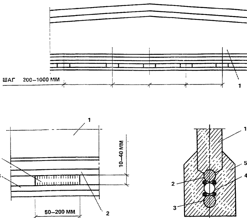
Рис. 12. Усиление растянутой зоны балок приваркой дополнительной арматуры через коротыши
