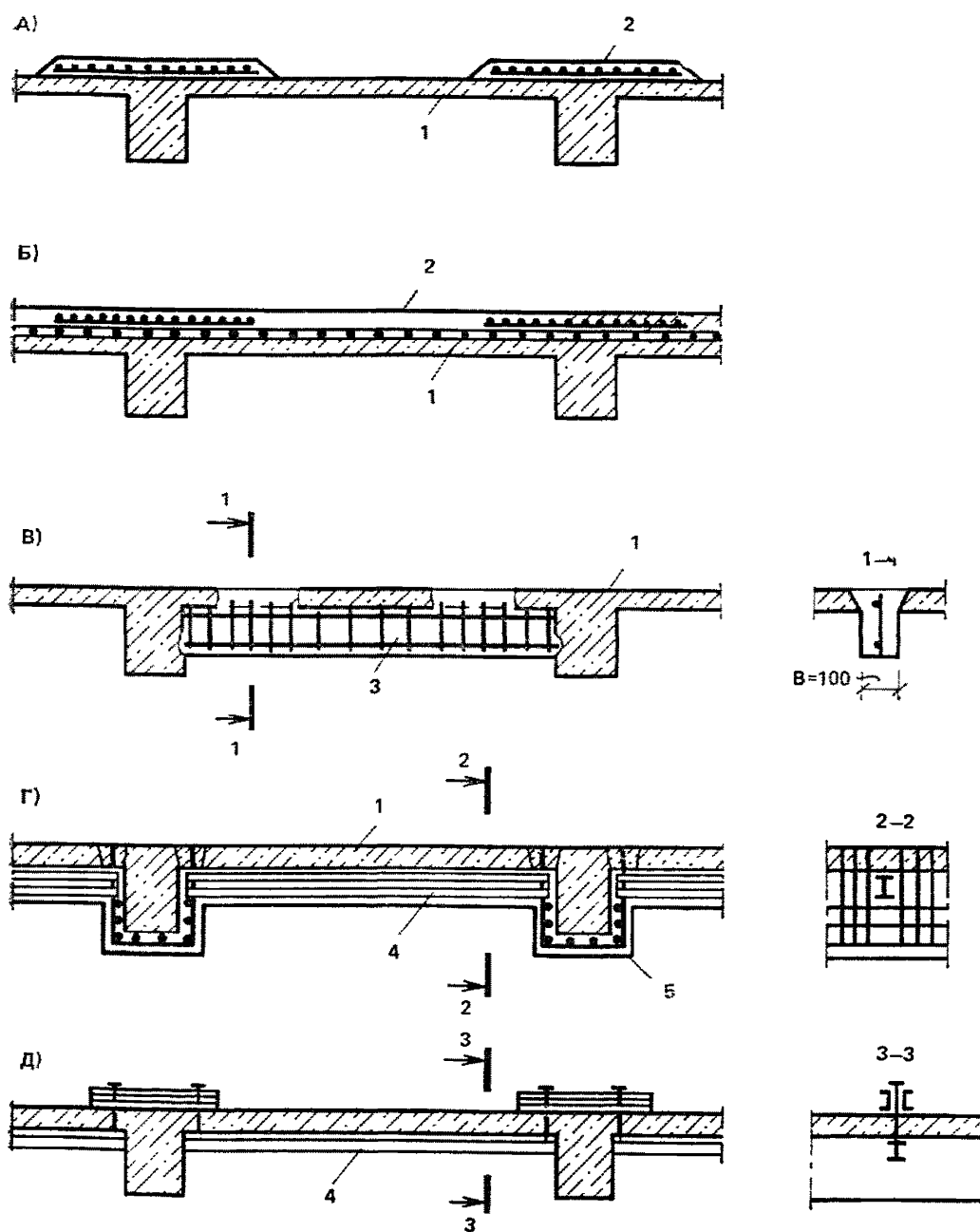
Рис. 2. Усиление плит железобетонных монолитных перекрытий
