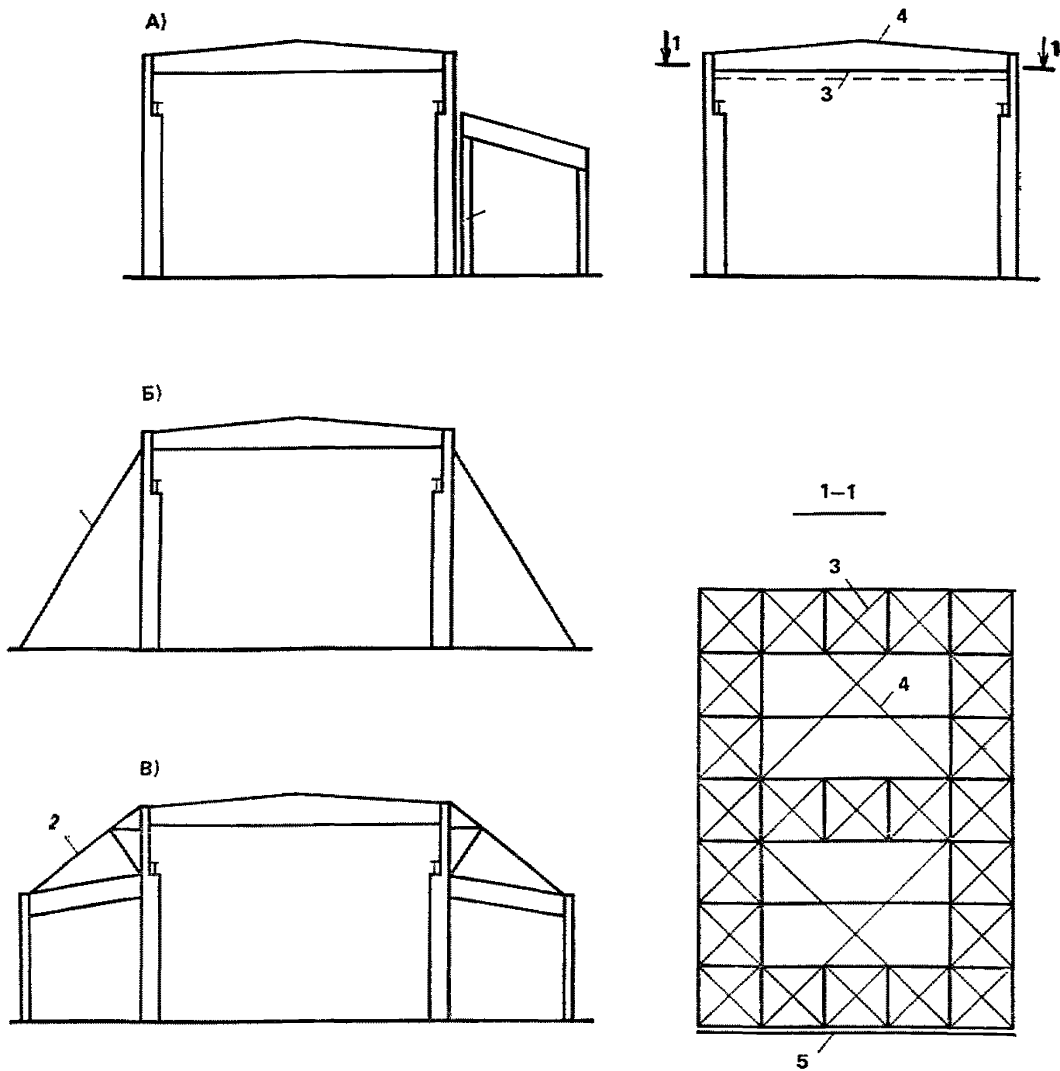
Рис. 63. Схемы усиления колонн каркаса изменением статической схемы
