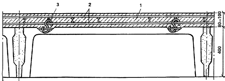
Рис. 3. Усиление ребристых плит перекрытий многоэтажных производственных зданий 1 — замоноличивающий слой бетона; 2 — дополнительная арматура; 3 — связующая шпилька
