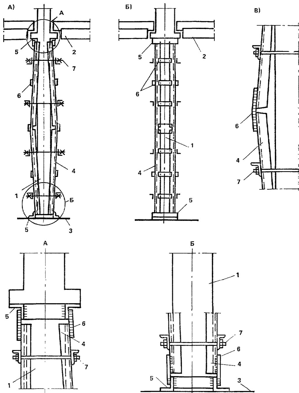
Рис. 23. Усиление колонн стальной облоймой (с преднапряжением, стягиванием ветвей или подклинкой)
