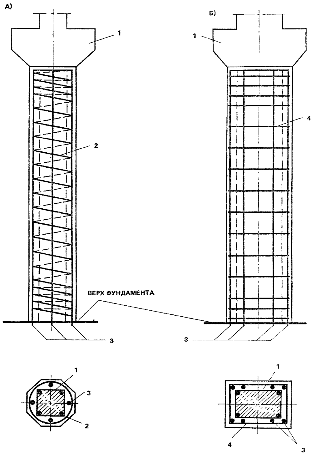
Рис. 21. Усиление колонн железобетонными обоймами
