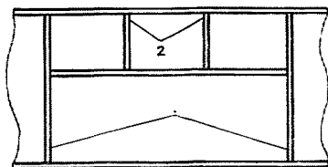
Рис. 40. Усиление стенки балки дополнительными ребрами
