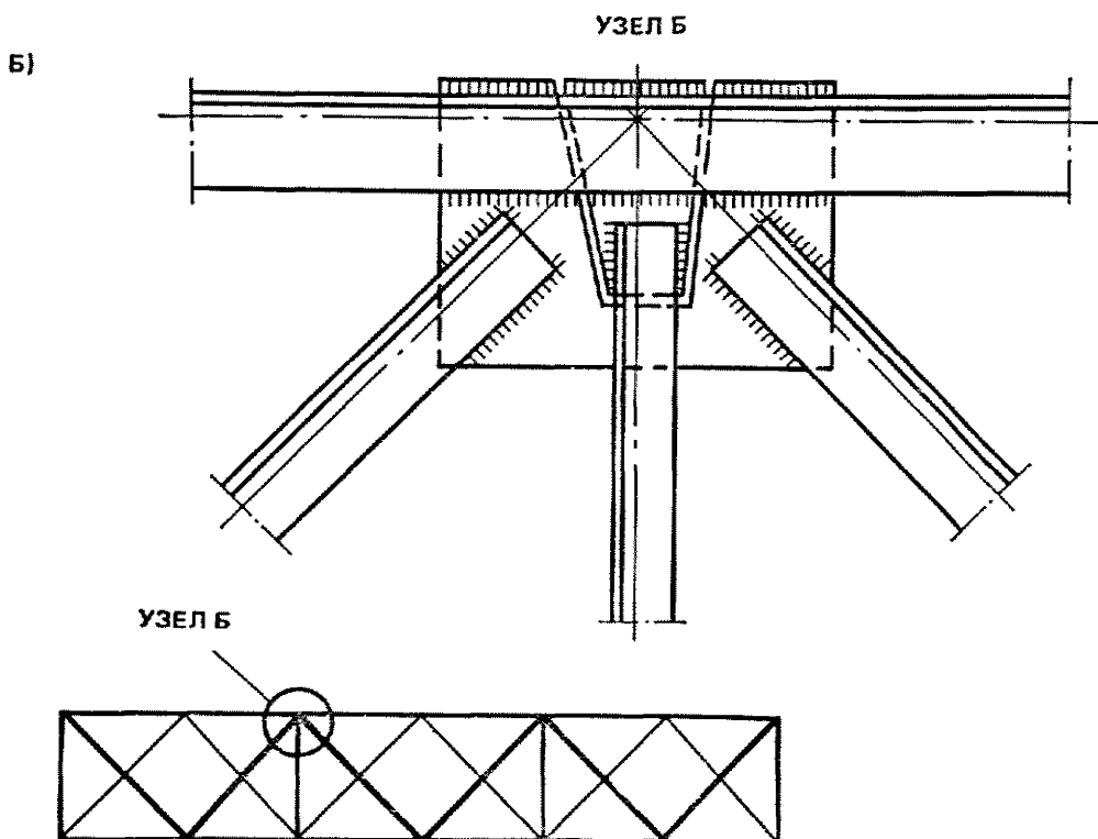
Рис. 56. Примеры восстановления А — колонны — заменой поврежденных частей; Б — ферм — устройством второй решетки (жирными линиями показаны новые раскосы и фасонки)
