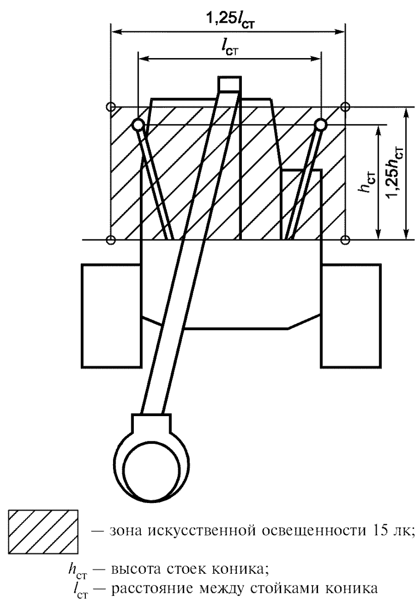
Рисунок Б.2 — Трелевка леса бесчокерная
