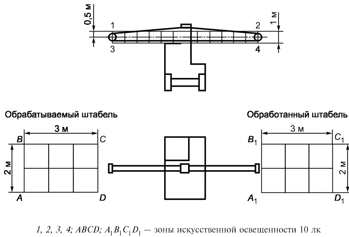
Рисунок Б.4 — Обрезка сучьев машинная
