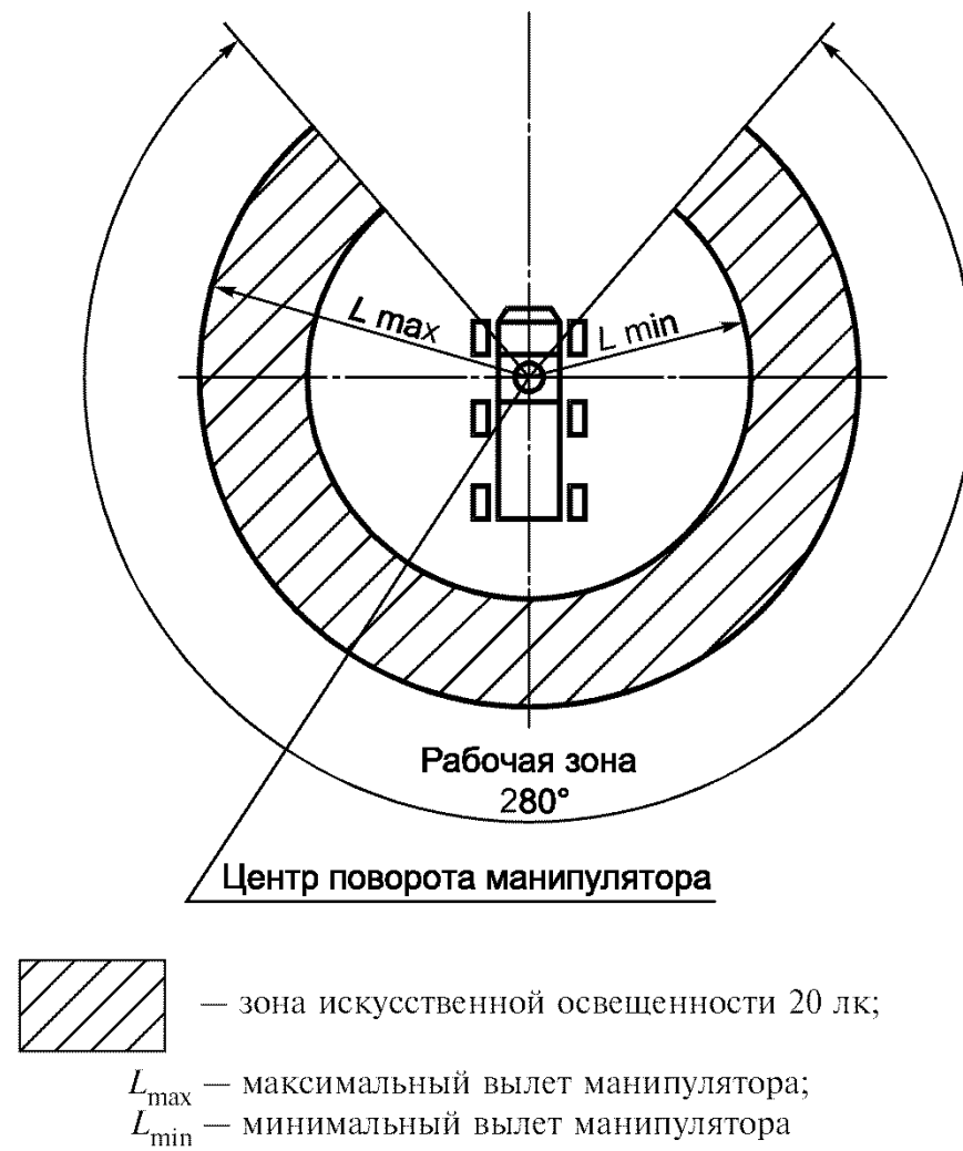
Рисунок Б.5 — Погрузочно-транспортные машины
