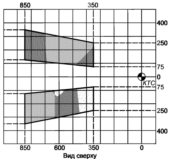
Рисунок 3 — Зоны расположения педалей двустороннего действия
