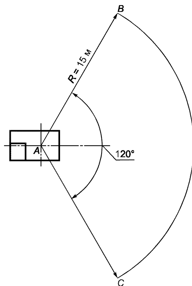
Рисунок Б.2 — Трелевка леса бесчокерная
